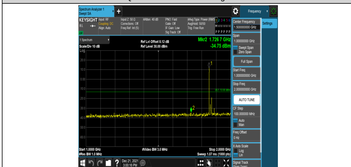
Band2-20MHz-QPSK-18700-1RB#0-Range4:1000~2000MHz
