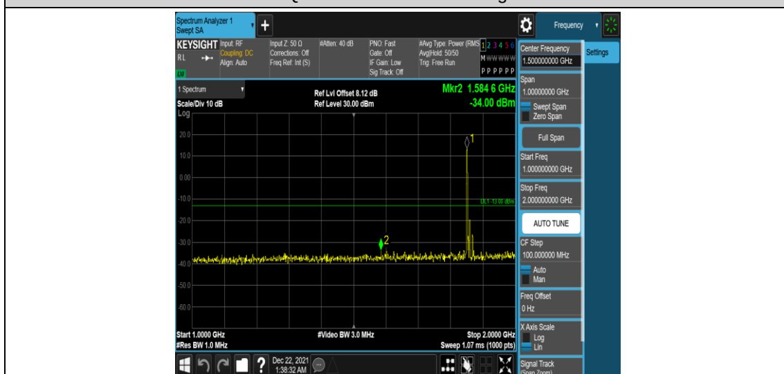
Band25-10MHz-QPSK-26090-1RB#0-Range4:1000~2000MHz
