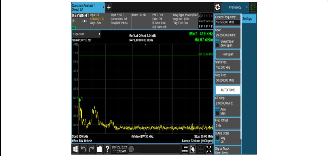
Band25-5MHz-QPSK-26365-1RB#0-Range2:0.15~30MHz
