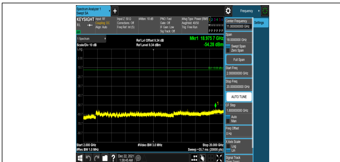
Band25-10MHz-QPSK-26090-1RB#0-Range5:2000~20000MHz
