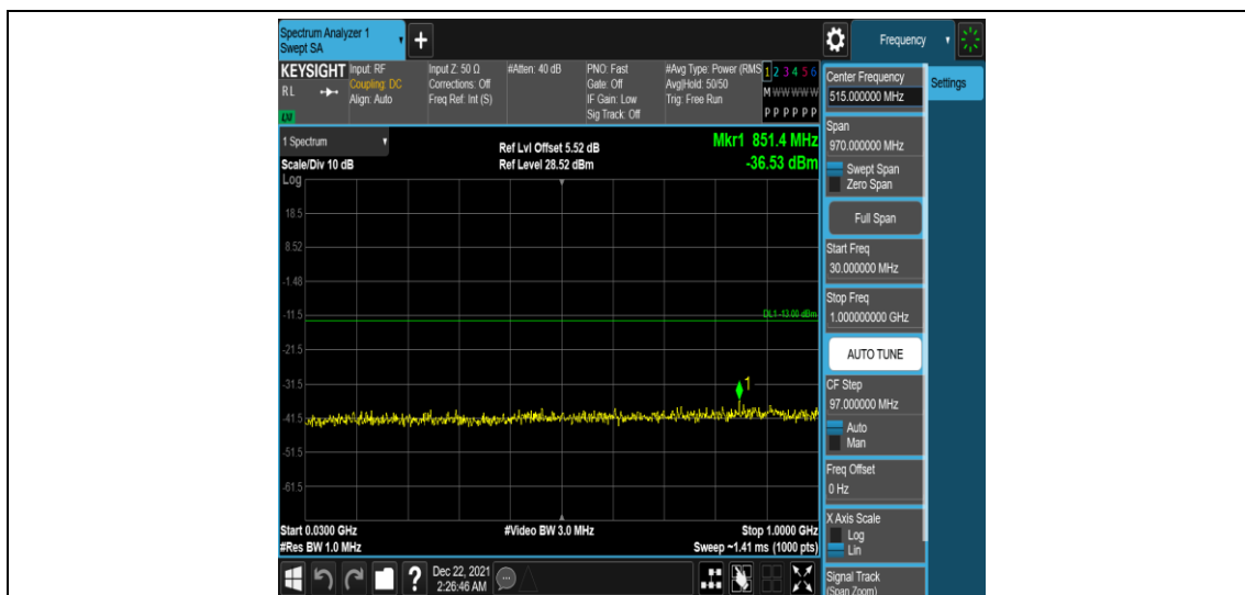
Band25-20MHz-QPSK-26365-1RB#0-Range3:30~1000MHz
