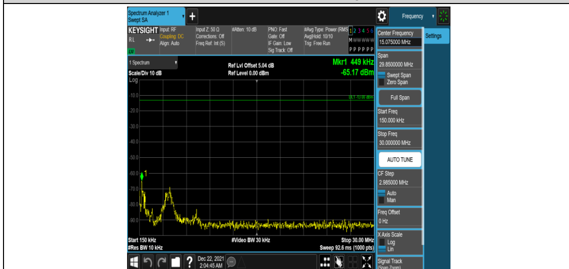
Band25-15MHz-QPSK-26615-1RB#0-Range2:0.15~30MHz
