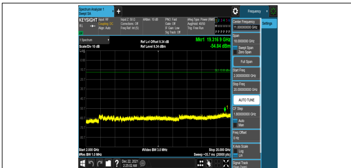
Band25-20MHz-QPSK-26140-1RB#0-Range5:2000~20000MHz
