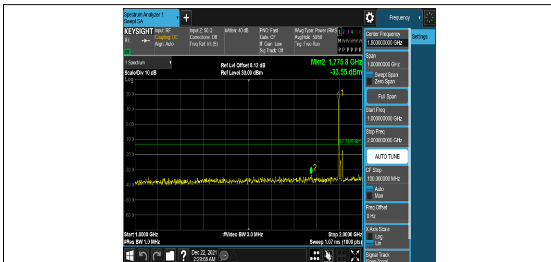
Band25-20MHz-QPSK-26590-1RB#0-Range4:1000~2000MHz
