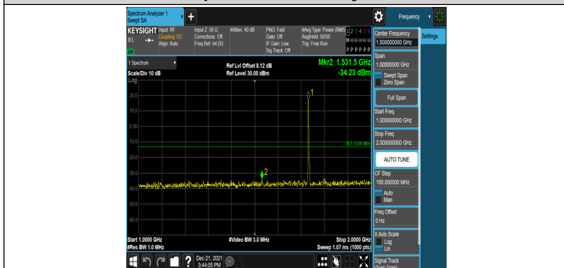
Band4-3MHz-QPSK-20175-1RB#0-Range4:1000~2000MHz
