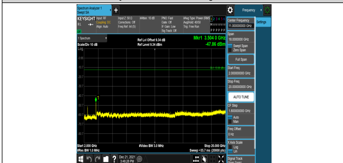
Band4-3MHz-QPSK-20385-1RB#0-Range5:2000~20000MHz
