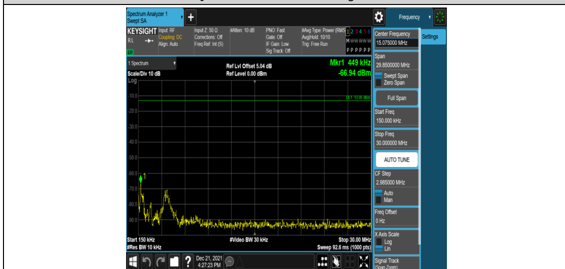
Band4-10MHz-QPSK-20175-1RB#0-Range2:0.15~30MHz
