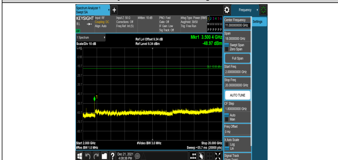
Band4-5MHz-QPSK-20375-1RB#0-Range5:2000~20000MHz
