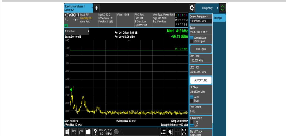
Band5-5MHz-QPSK-20525-1RB#0-Range2:0.15~30MHz
