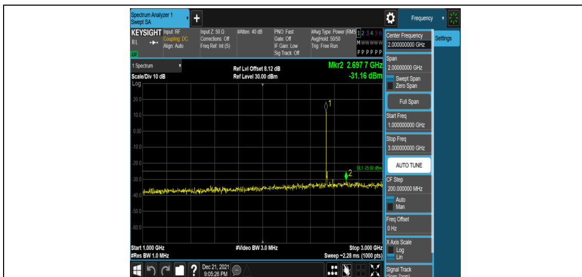
Band7-10MHz-QPSK-21100-1RB#0-Range4:1000~3000MHz
