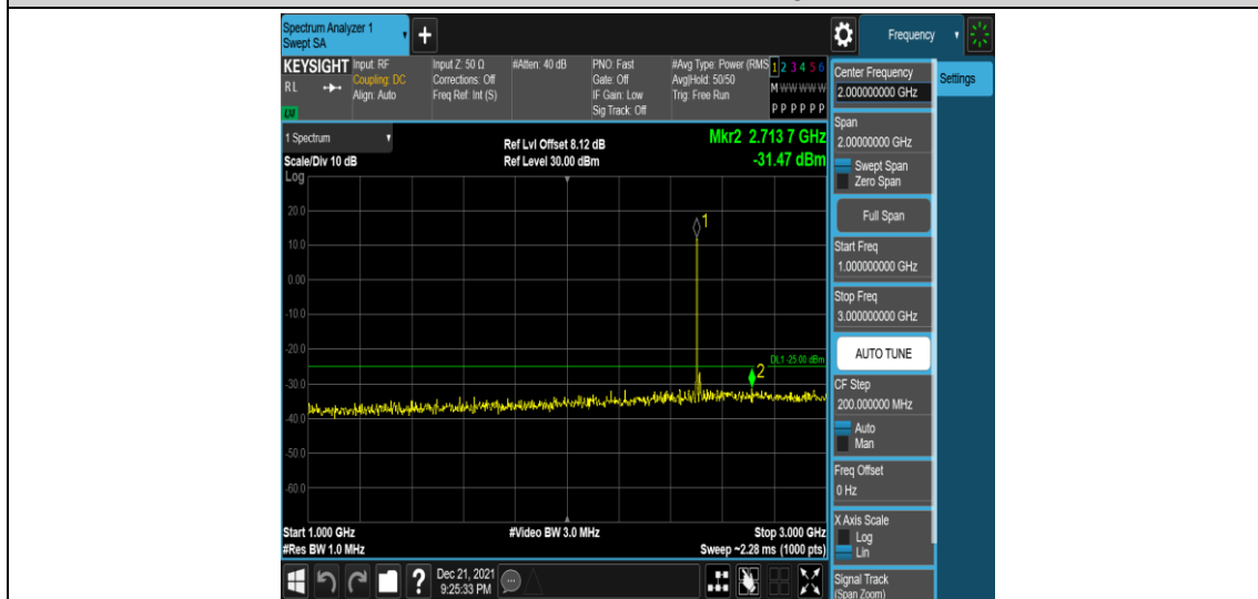
Band7-15MHz-QPSK-20825-1RB#0-Range4:1000~3000MHz
