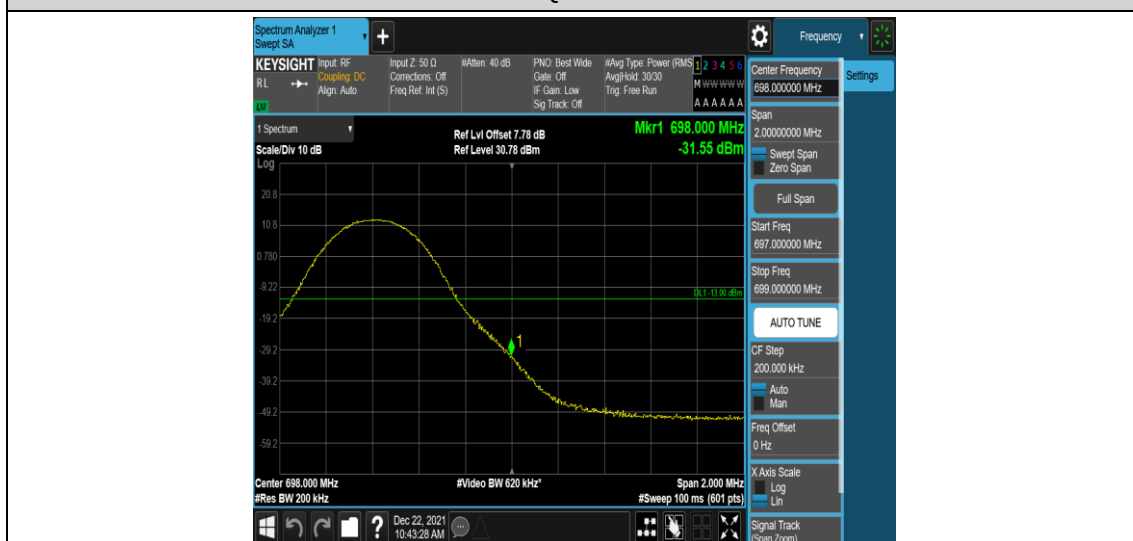
Band71-10MHz-QPSK-133422-1RB#49
