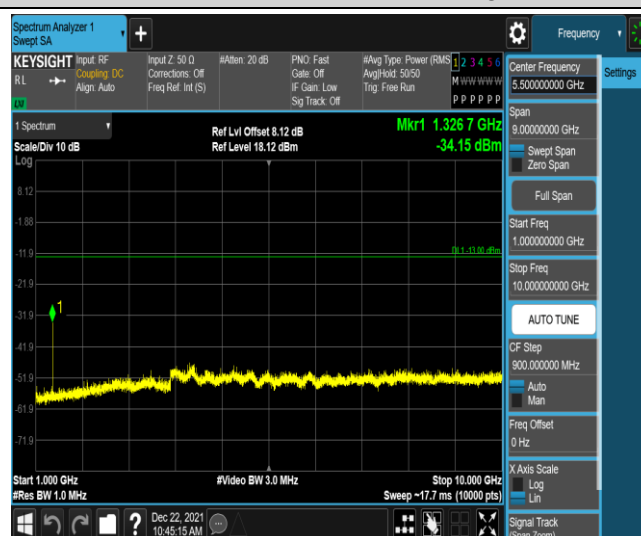
Band71-10MHz-QPSK-133172-1RB#0-Range4:1000~10000MHz
