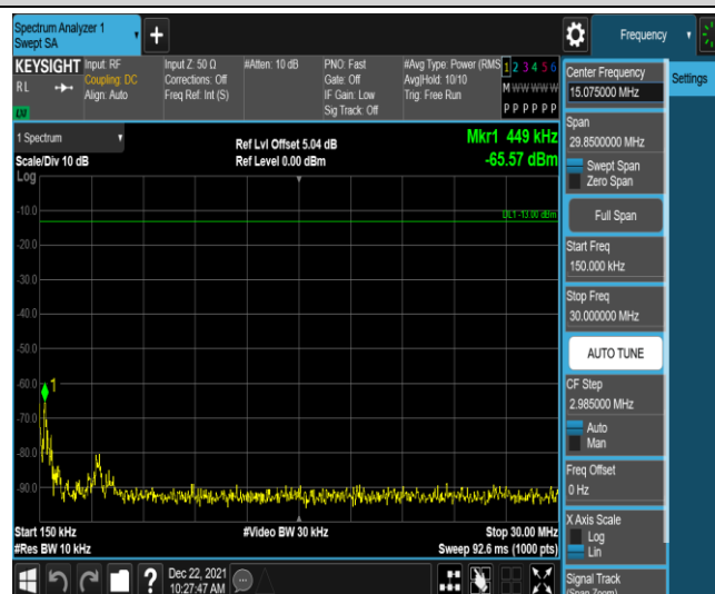
Band71-5MHz-16QAM-133447-1RB#0-Range2:0.15~30MHz
