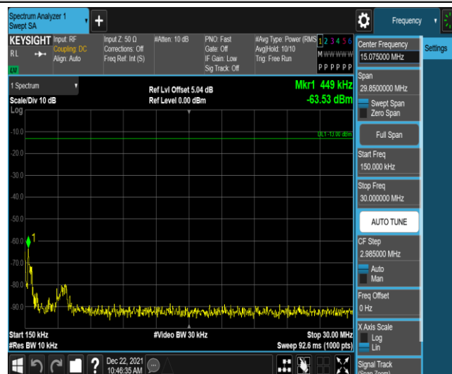
Band71-10MHz-QPSK-133297-1RB#0-Range2:0.15~30MHz
