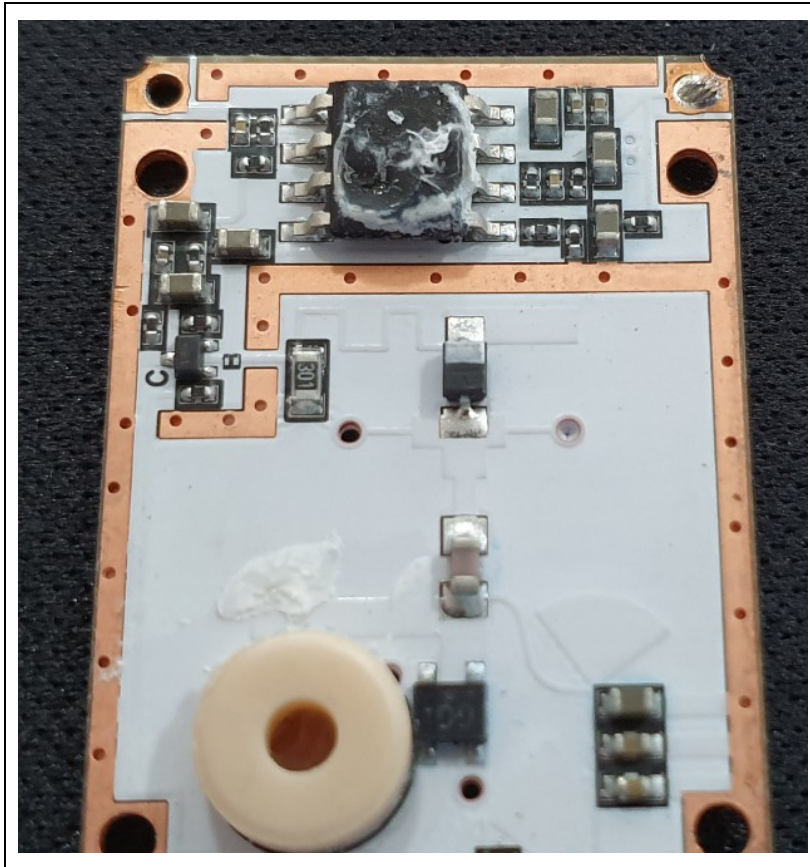
<Antenna>
