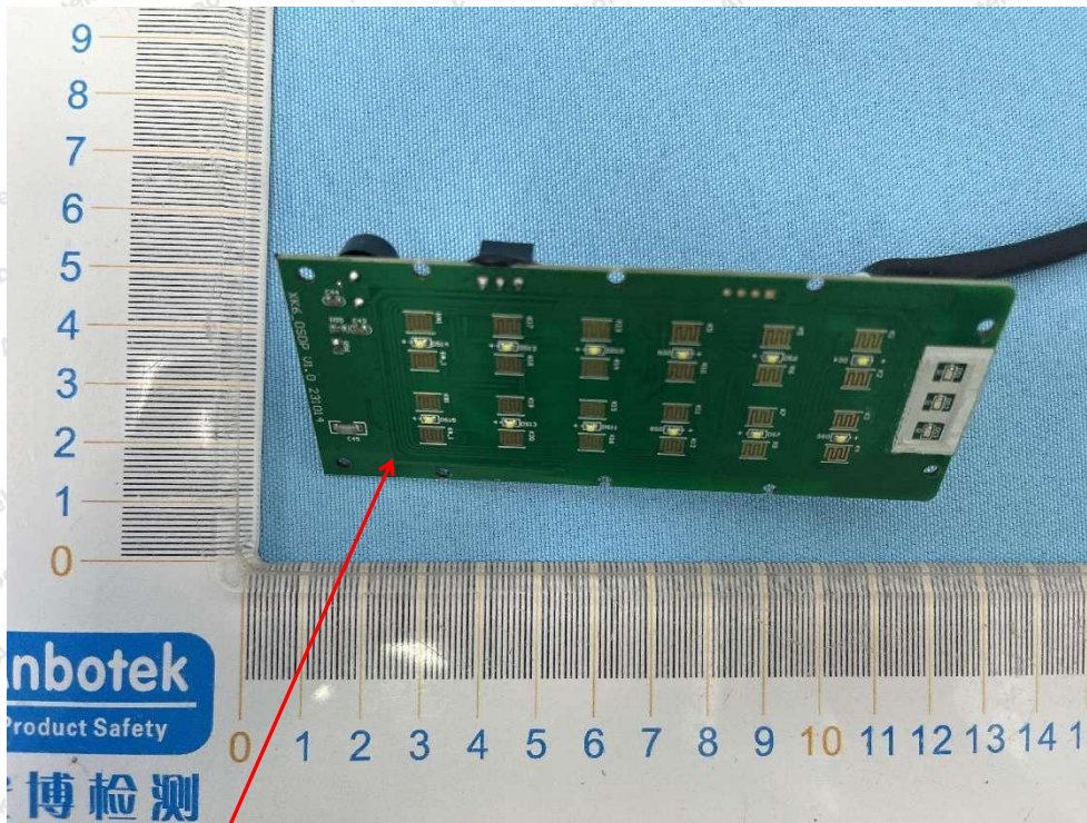
13.56MHz ANT
