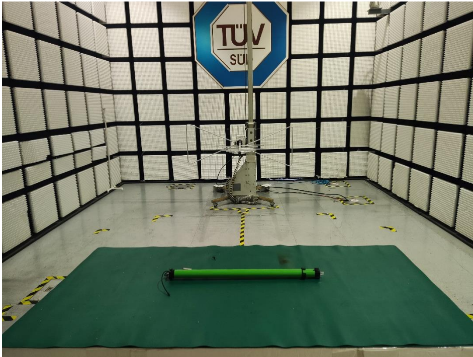
30MHz ~ 1GHz DC mode
