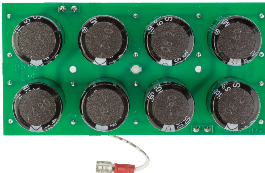
Figure 15 – HVF1kW_V3 top side
