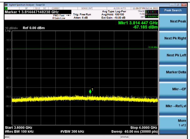
3600-4000 MHz Ch 39
