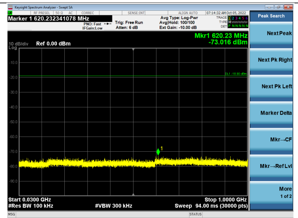
30-1000 MHz Ch 17
