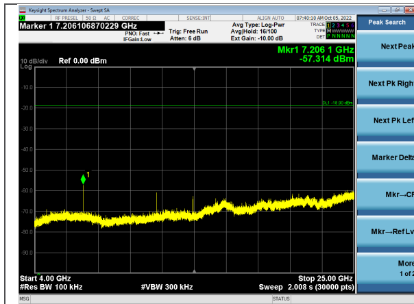
4000-25000 MHz Ch 37
