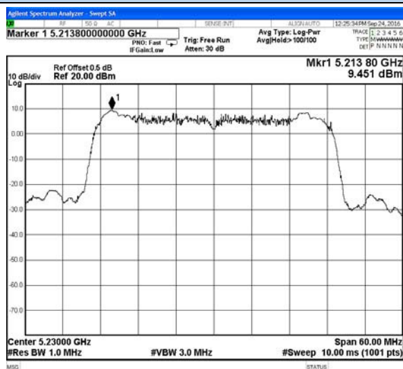
Chain 0-5230MHz
