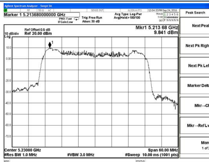
Chain 1-5230MHz
