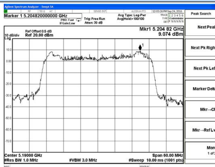
Chain 1-5190MHz
