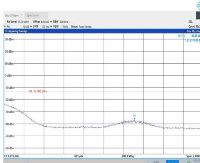
Band25-20MHz-16QAM-26590-1RB#99
