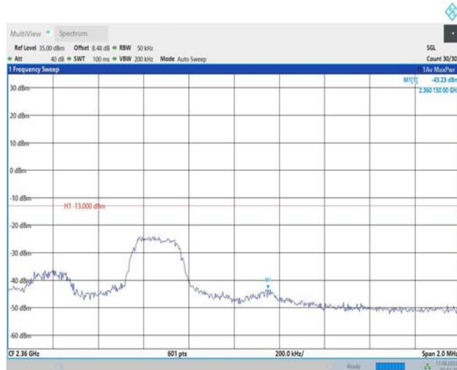
Band40-5MHz-QPSK-39225-1RB#24
