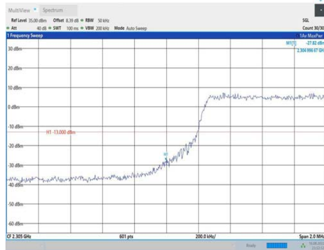
Band40-5MHz-QPSK-38775-1RB#0
