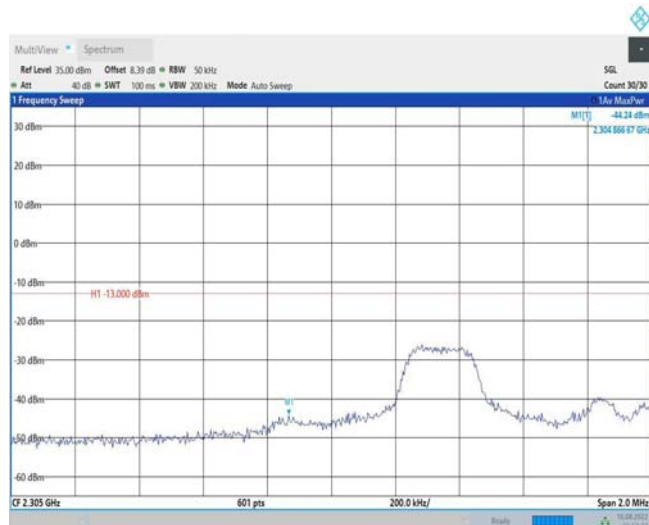
Band40-5MHz-QPSK-38725-25RB#0
