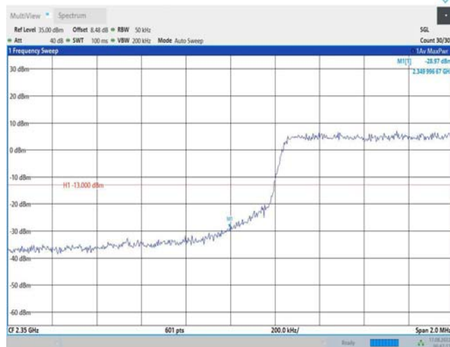
Band40-5MHz-QPSK-39225-1RB#0
