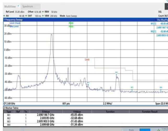
Band41-5MHz-16QAM-41565-1RB#24
