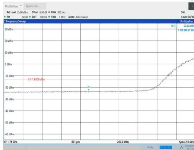
Band66-20MHz-QPSK-132572-1RB#0
