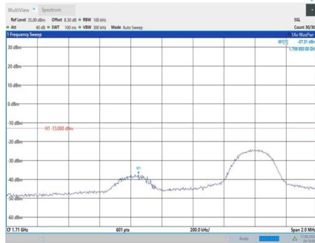
Band66-10MHz-QPSK-132022-50RB#0
