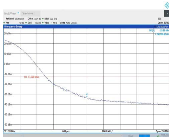
Band66-20MHz-QPSK-132572-100RB#0
