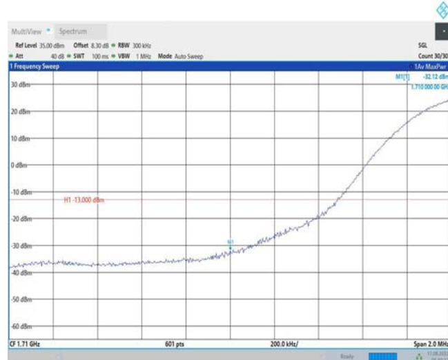
Band66-20MHz-16QAM-132072-1RB#99
