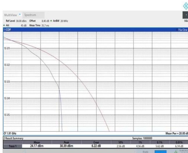
Band25-10MHz-QPSK-26640-50RB#0
