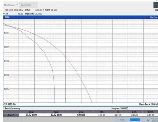
Band25-3MHz-QPSK-26365-15RB#0
