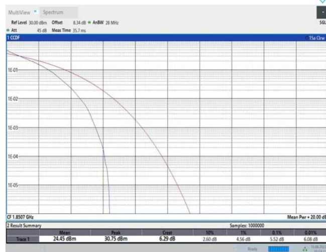
Band25-1.4MHz-QPSK-26365-1RB#0
