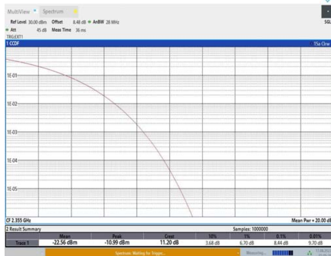
Band40-10MHz-QPSK-39200-50RB#0
