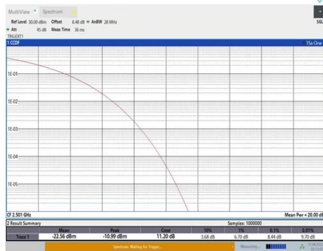
Band41-10MHz-QPSK-39700-50RB#0
