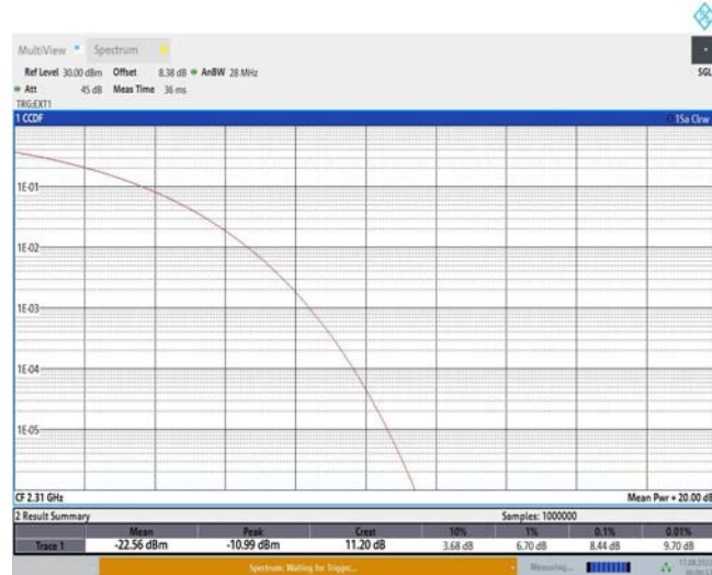
Band40-5MHz-QPSK-38775-1RB#0
