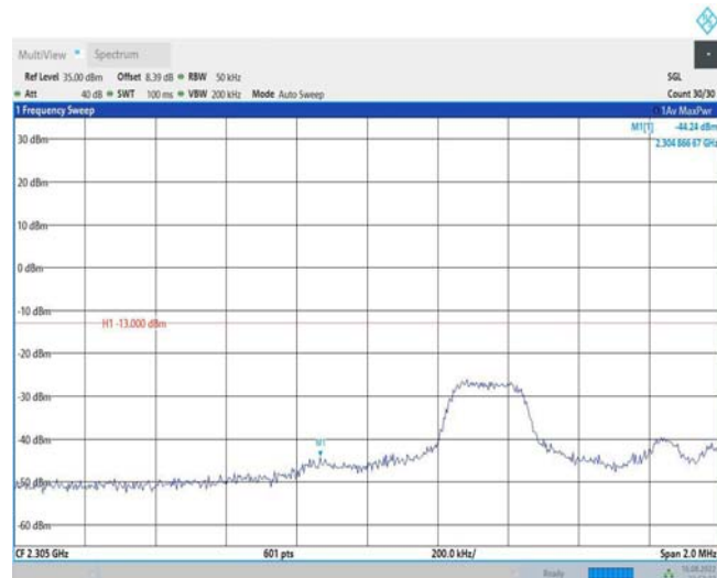
Band40-5MHz-QPSK-38725-25RB#0
