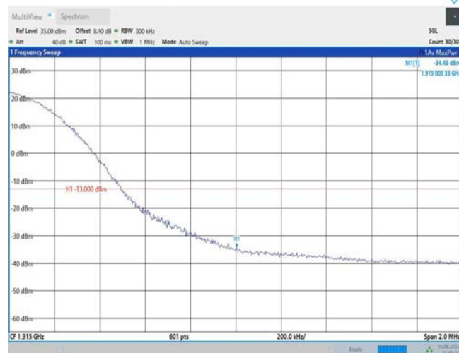
Band25-20MHz-QPSK-26590-100RB#0
