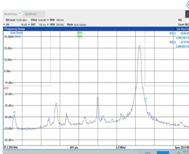
Band40-10MHz-QPSK-39200-50RB#0
