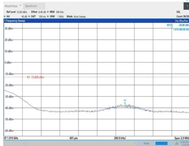
Band25-20MHz-QPSK-26590-1RB#99
