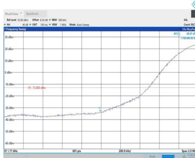
Band66-20MHz-QPSK-132072-1RB#99
