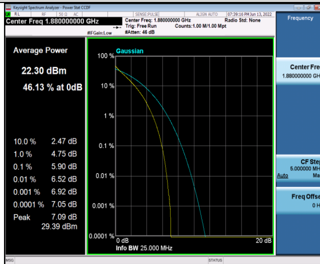
Band2-10MHz-QPSK-18800-50RB#0
