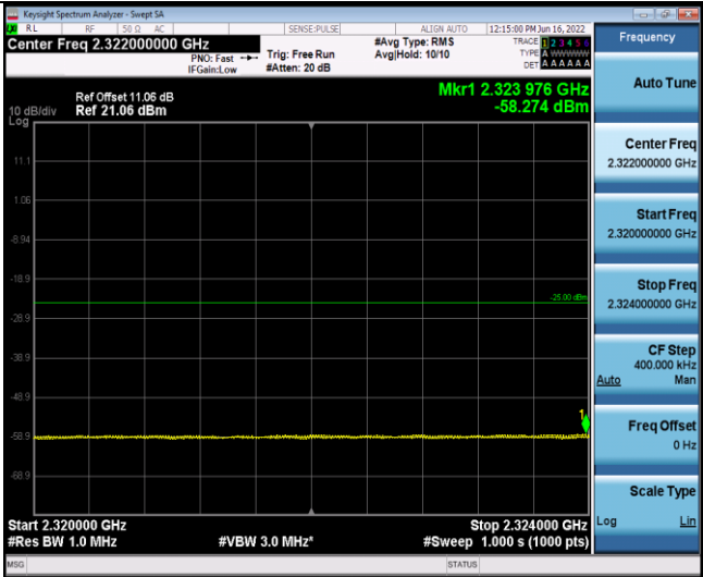
Band40-5MHz-QPSK-39200-25RB#0-Range7:2324~2328MHz
