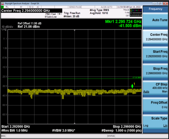
Band40-10MHz-QPSK-38750-50RB#0-Range5:2296~2300MHz
