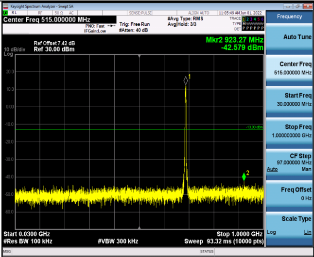
Band71-5MHz-QPSK-133447-25RB#0-Range2:1000~10000MHz
