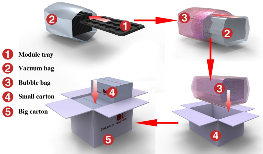
Figure43: packaging diagram
