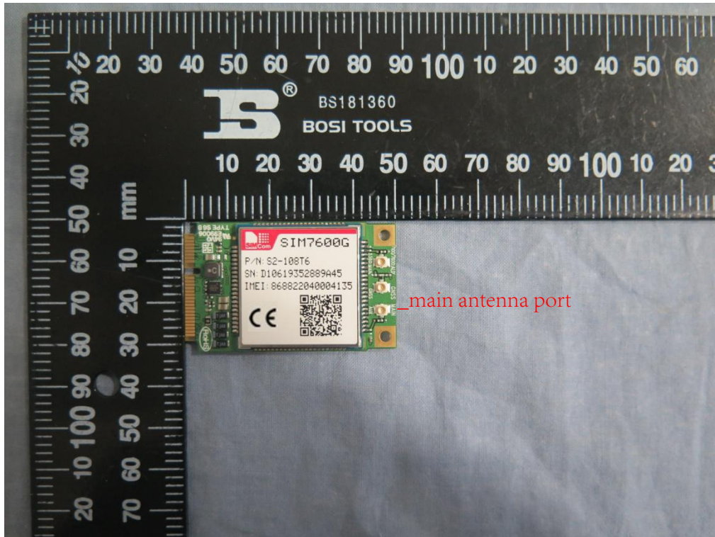
EUT FRONT
