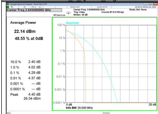
Band41_1_Q16_High
