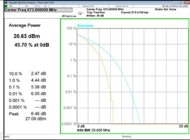
Band71_100_Q16_Low
