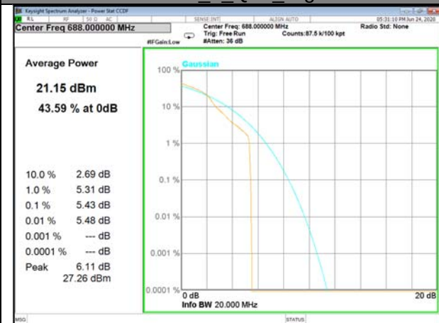
Band71_1_Q16_High
