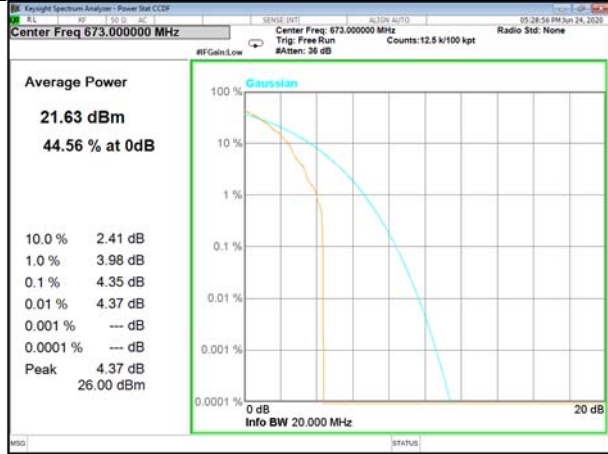
Band71_1_Q16_Low
