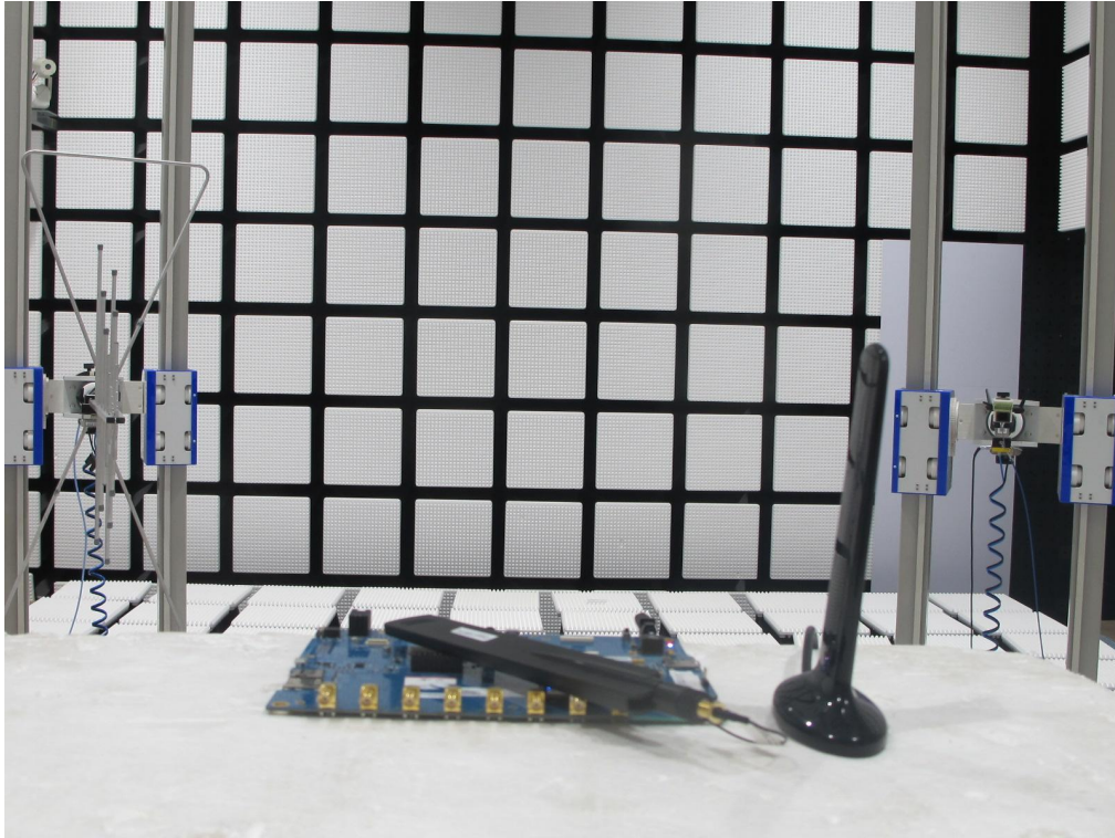
RSE_18GHz-20GHz
