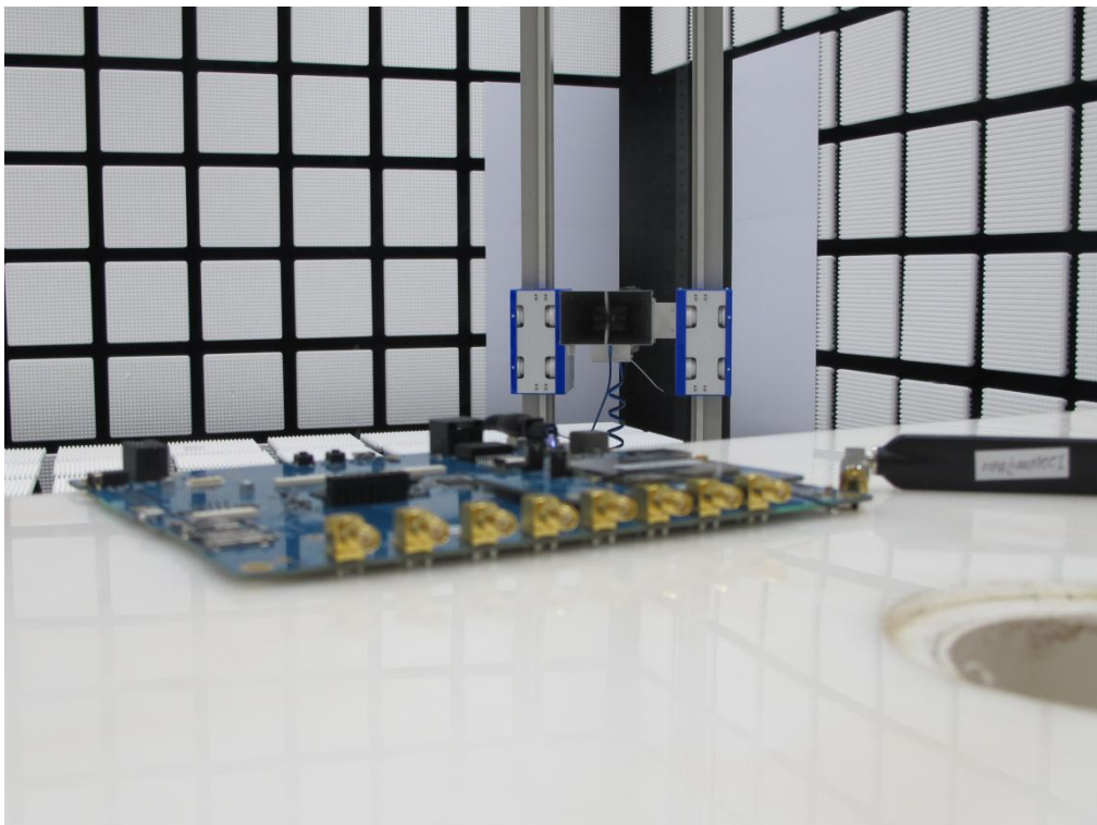
RSE (1GHz-18GHz)
