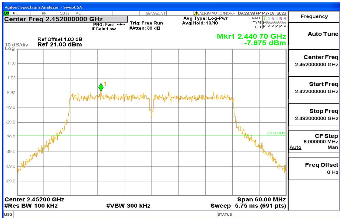
11n-HT40 Fig7
