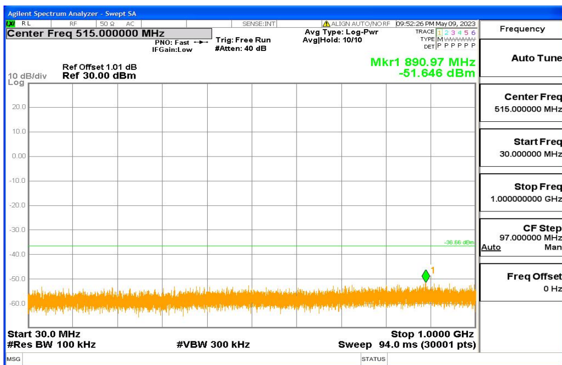
11n-HT20 Fig2
