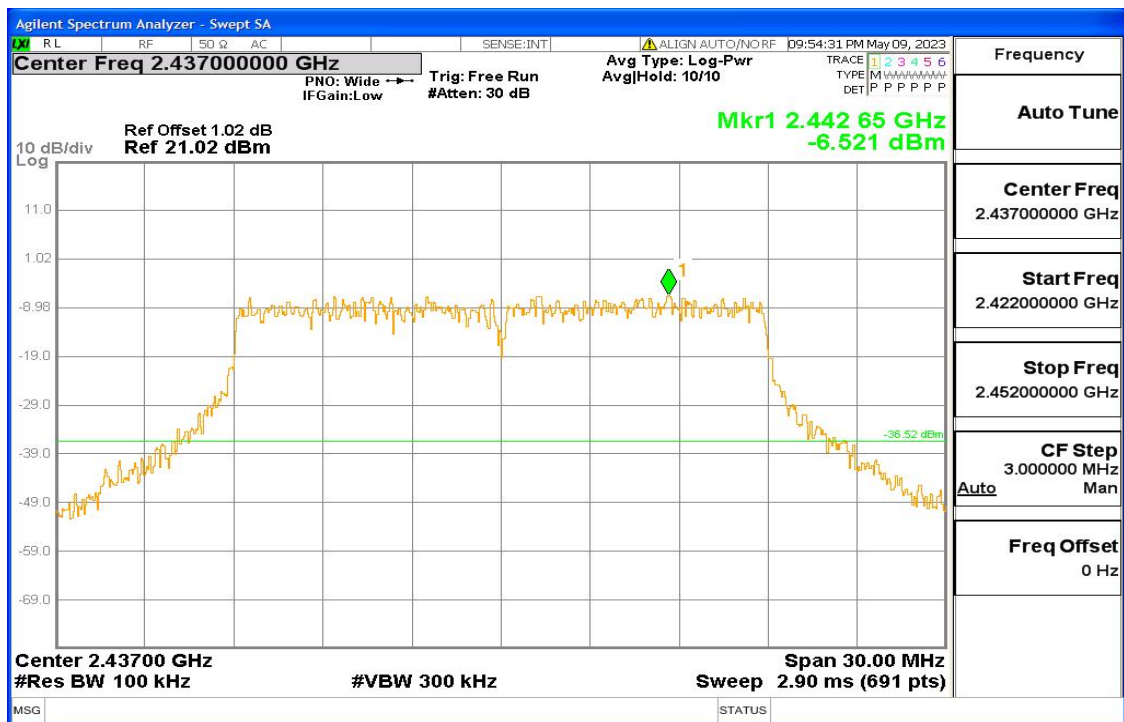
11n-HT20 Fig4
