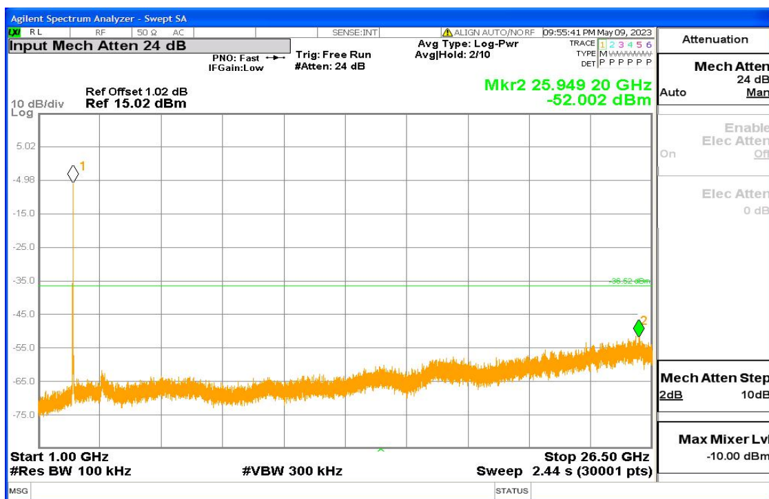
11n-HT20 Fig6
