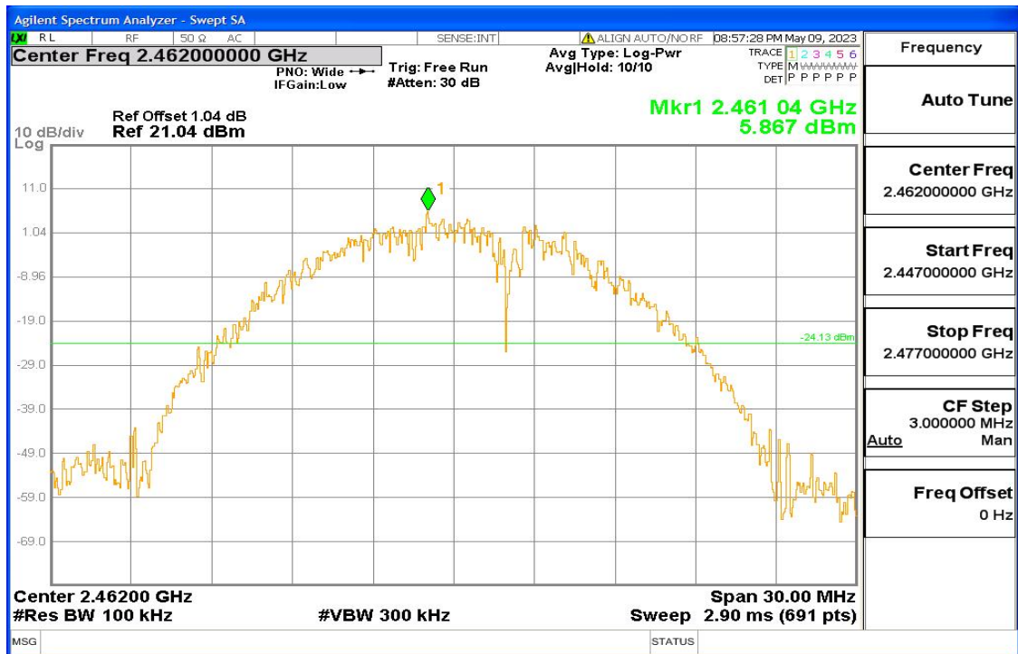
11b Fig7
