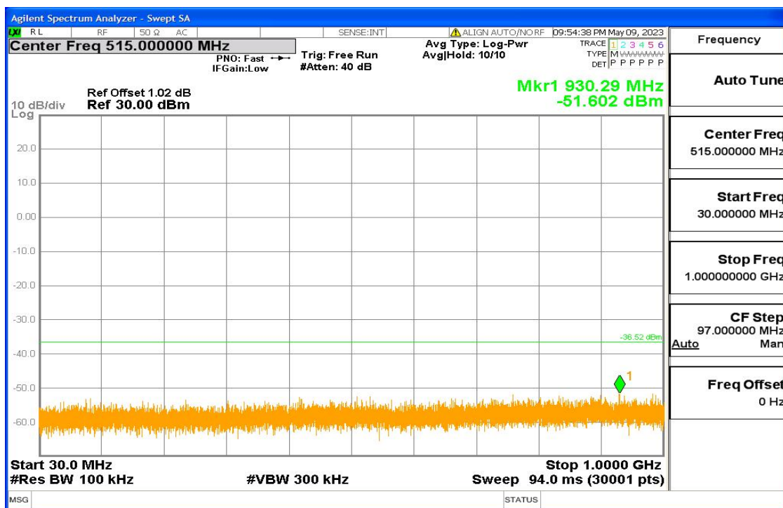
11n-HT20 Fig5
