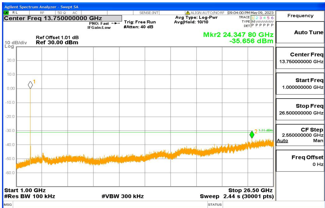
11g Fig3
