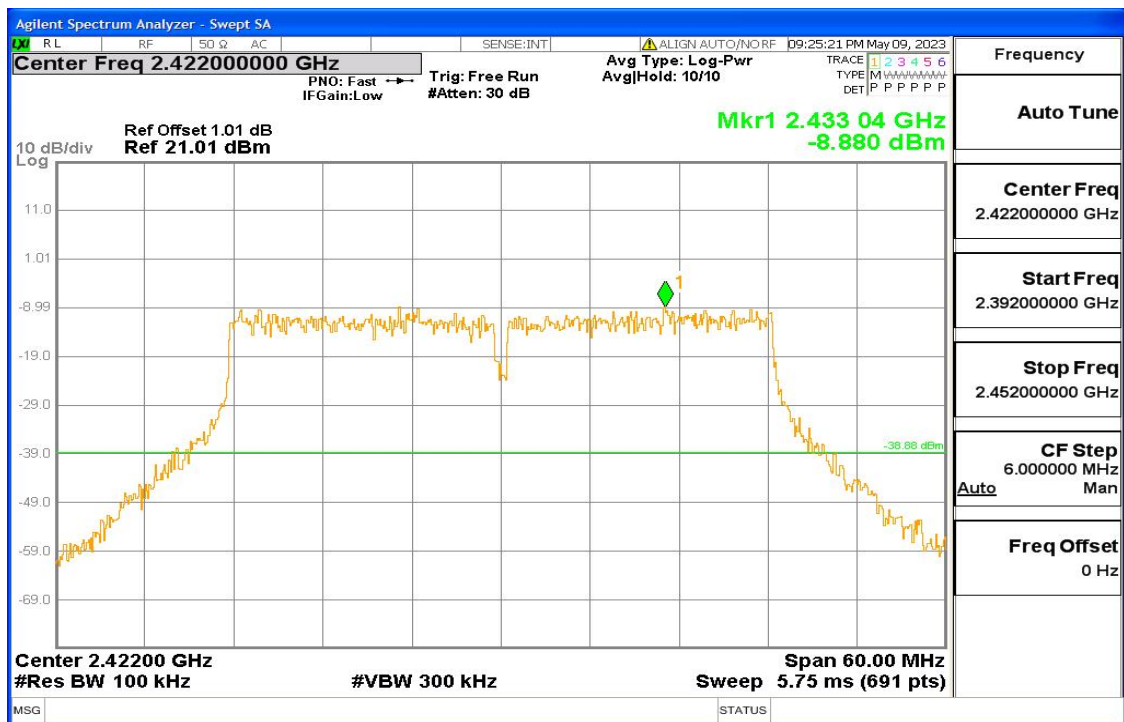
11n-HT40 Fig1
