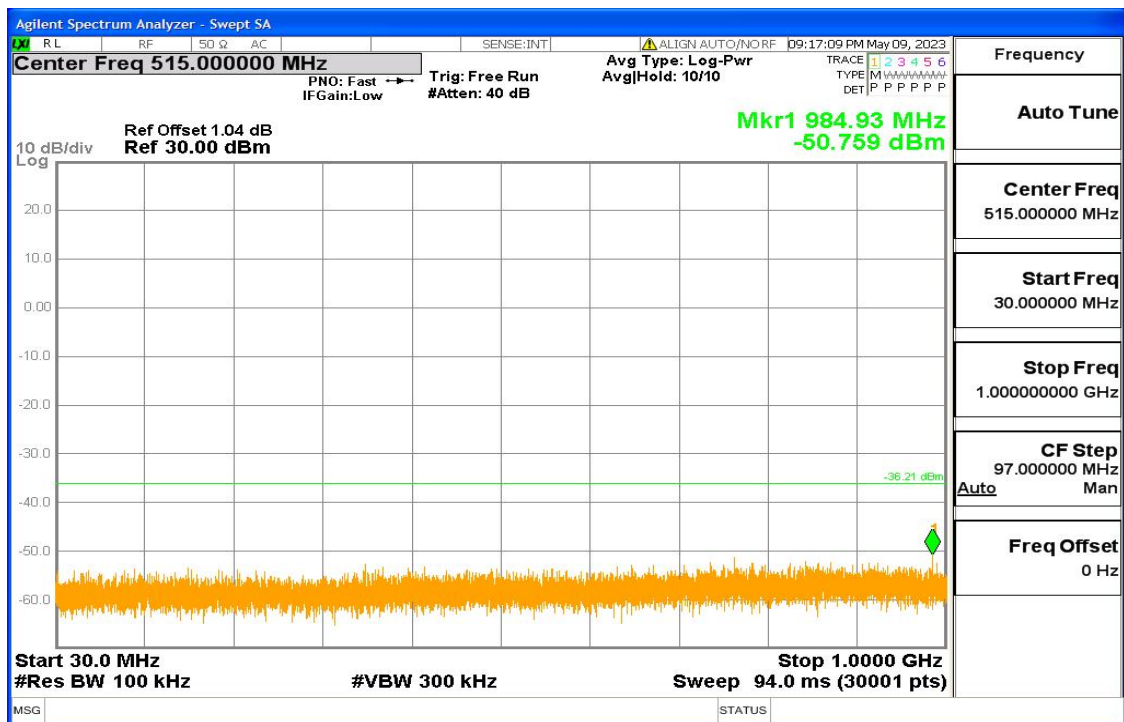
11n-HT20 Fig8
