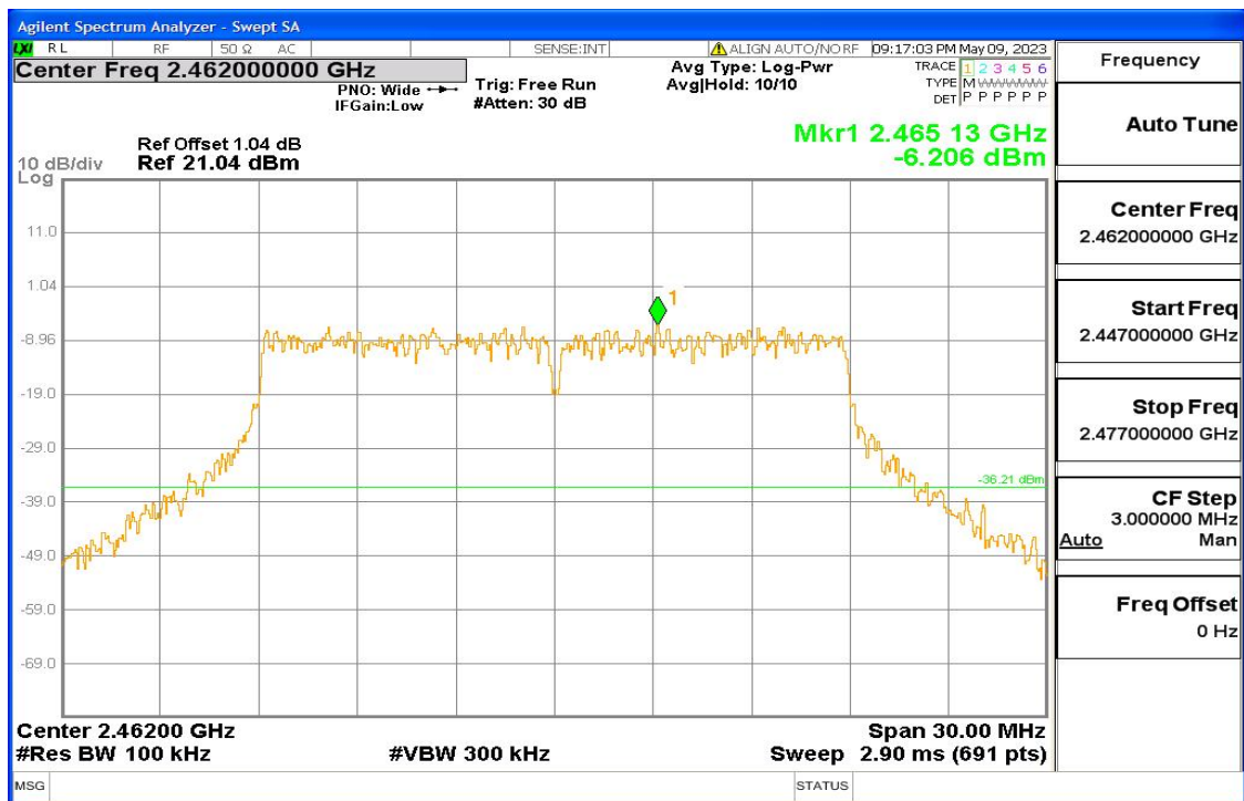
11n-HT20 Fig7
