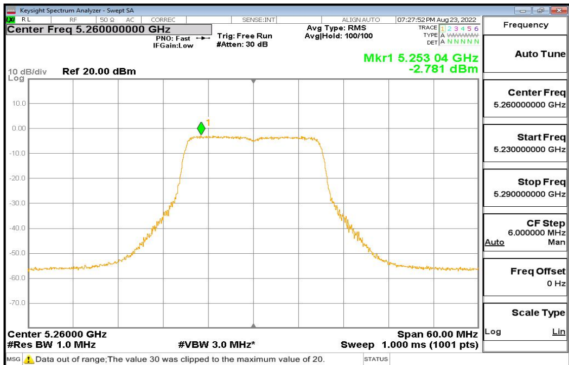
11n-20 Pic4
