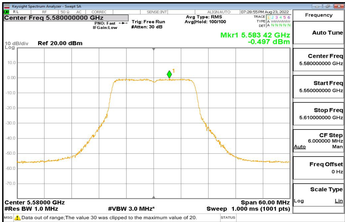
11n-20 Pic8
