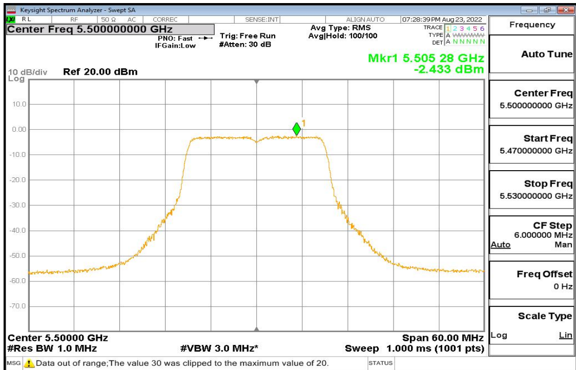
11n-20 Pic7
