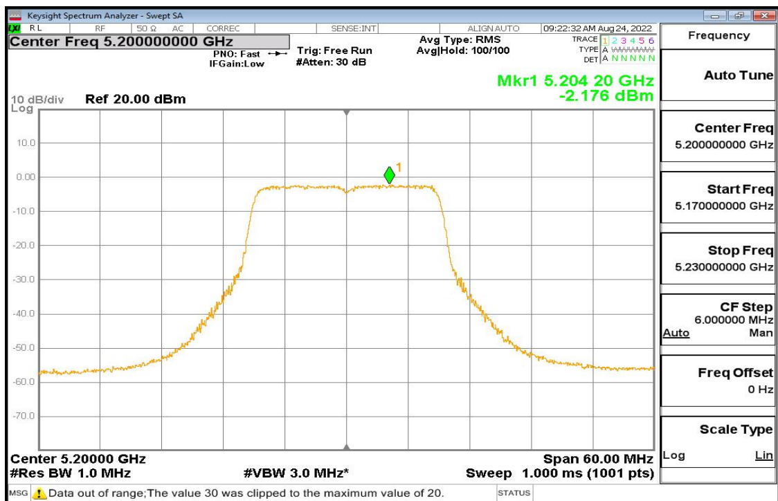
11n-20 Pic2
