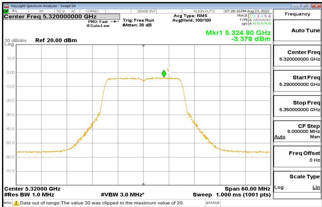
11n-20 Pic6
