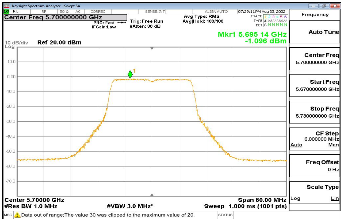
11n-20 Pic9
