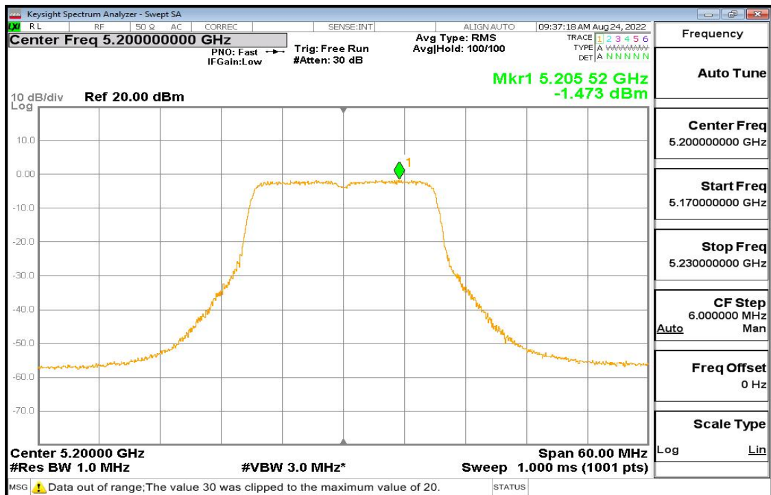
11ac-20 Pic2
