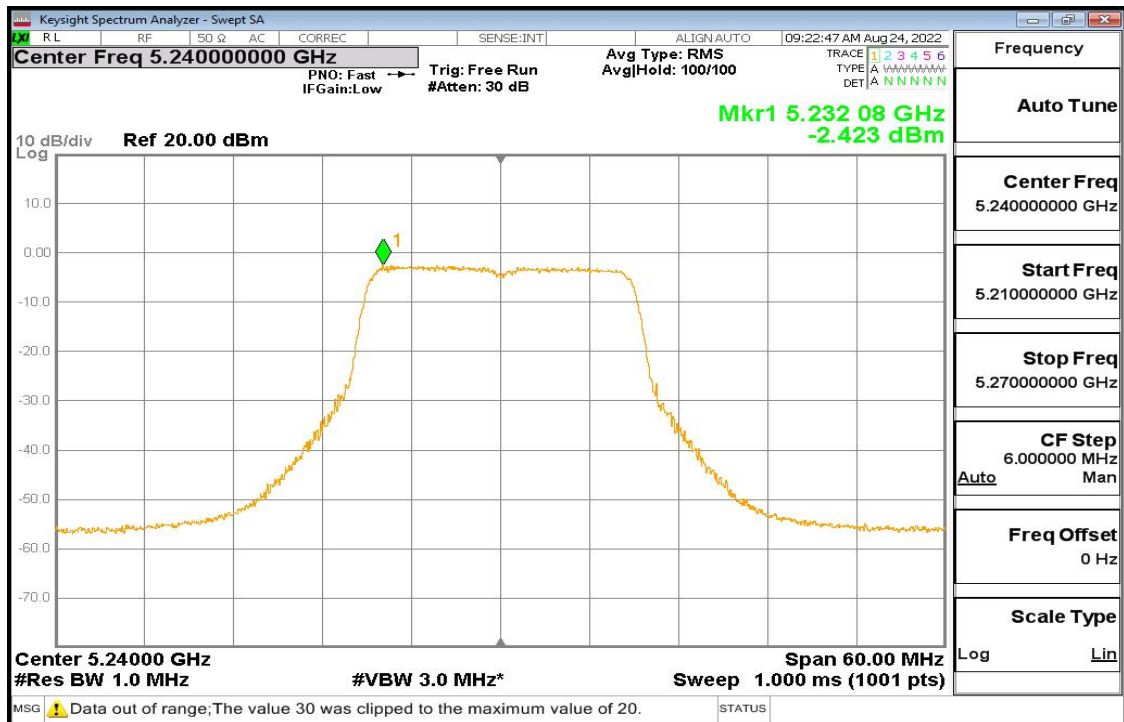
11n-20 Pic3
