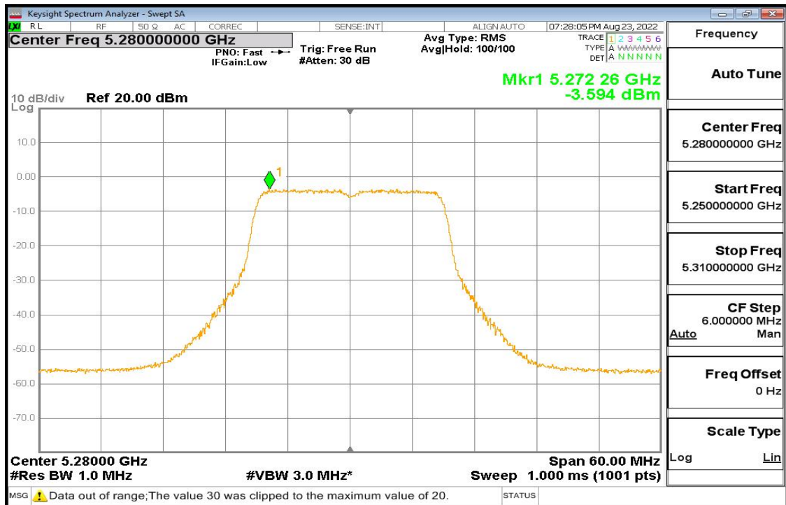
11n-20 Pic5
