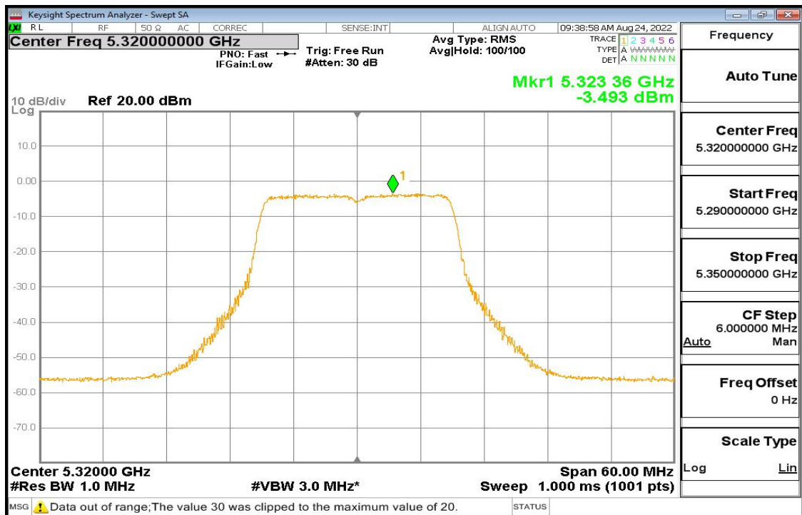
11ac-20 Pic6
