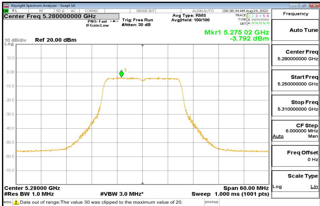
11ac-20 Pic5
