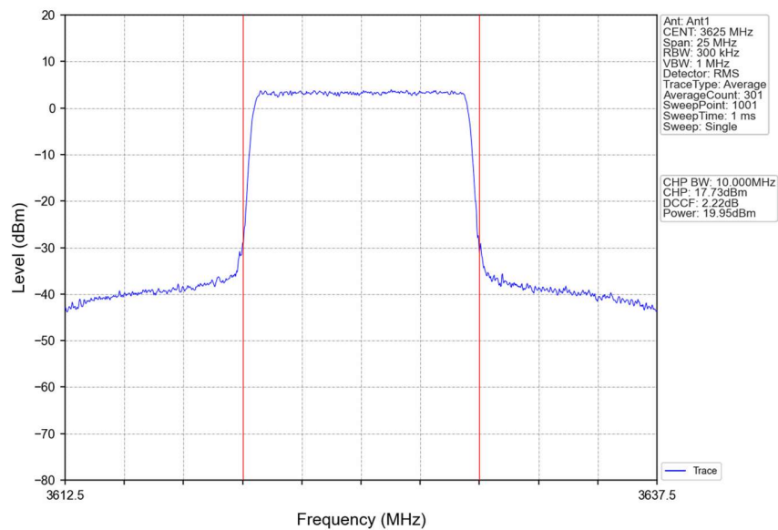
Band48_10MHz_QPSK_MCH_3625MHz_RB_50_0_NTNV
