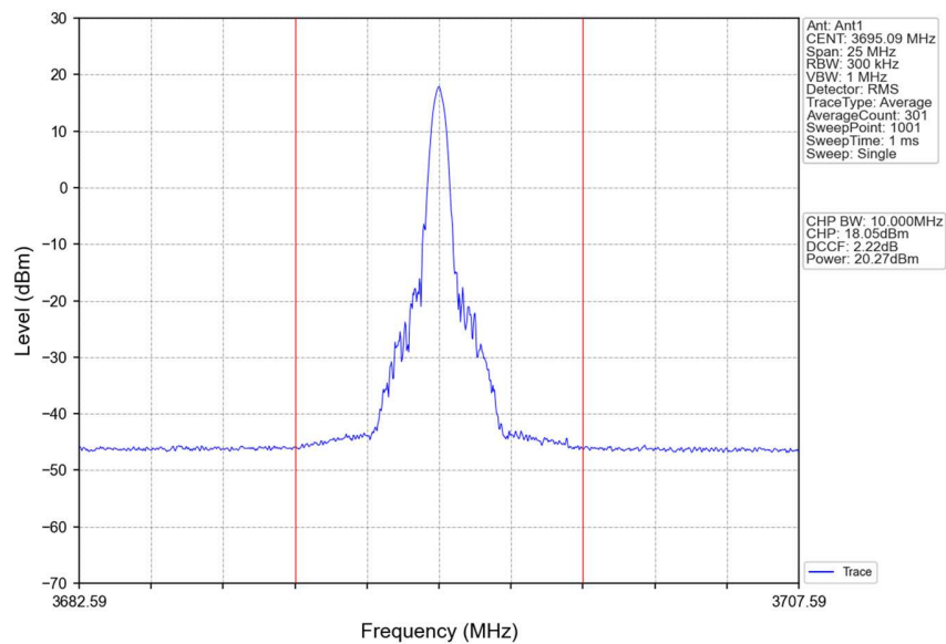
Band48_10MHz_16QAM_HCH_3695MHz_RB_1_49_NTNV
