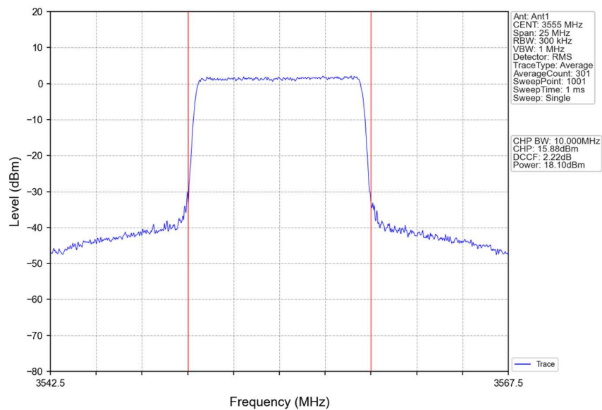
Band48_10MHz_16QAM_LCH_3555MHz_RB_50_0_NTNV
