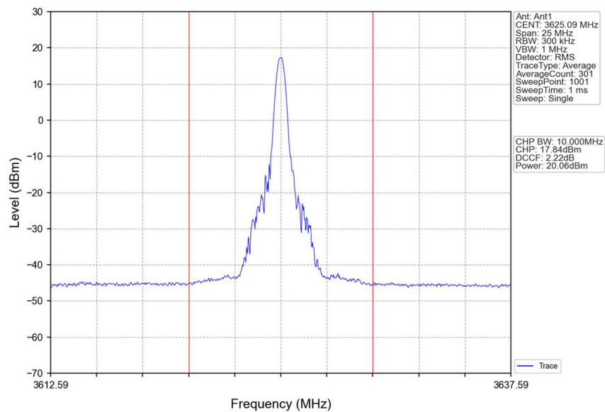
Band48_10MHz_16QAM_MCH_3625MHz_RB_1_25_NTNV
