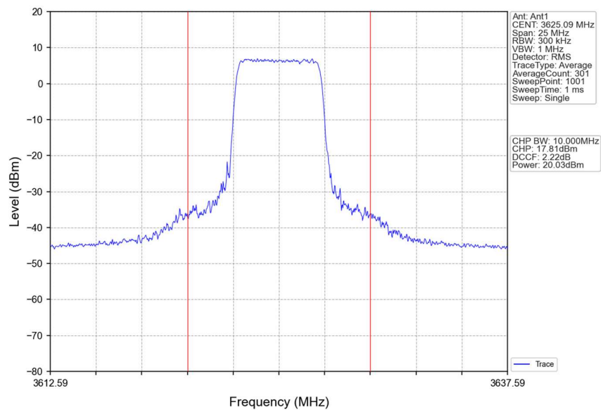
Band48_10MHz_QPSK_MCH_3625MHz_RB_25_13_NTNV
