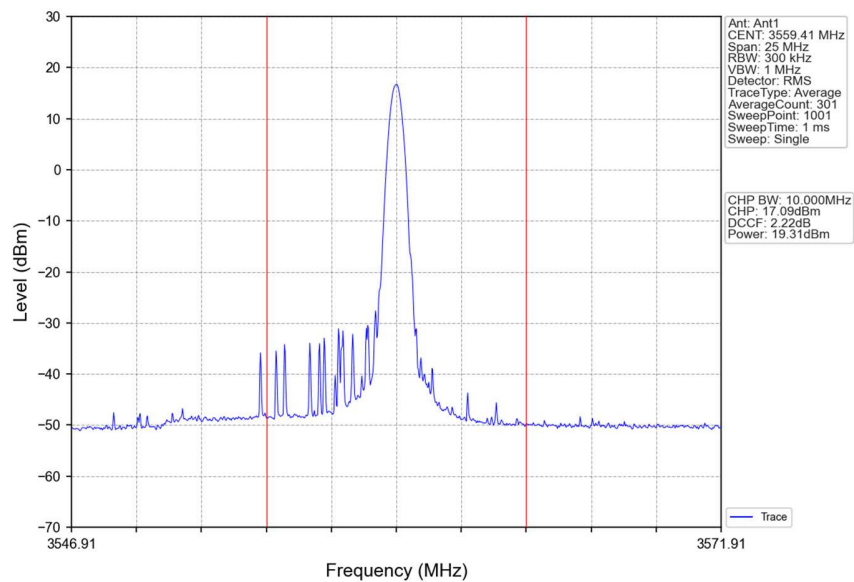
Band48_10MHz_16QAM_LCH_3555MHz_RB_1_49_NTNV
