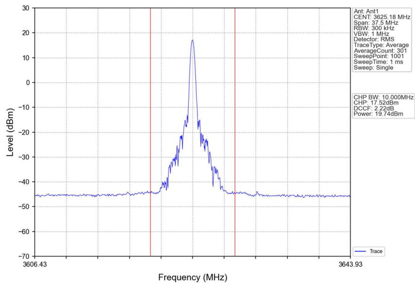
Band48_15MHz_QPSK_MCH_3625MHz_RB_1_74_NTNV
