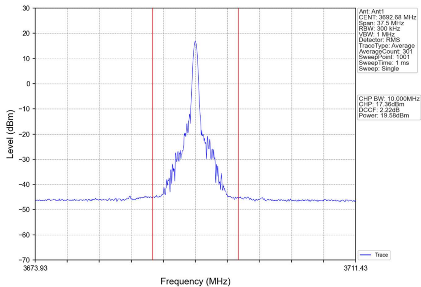
Band48_15MHz_QPSK_HCH_3692.5MHz_RB_1_38_NTNV
