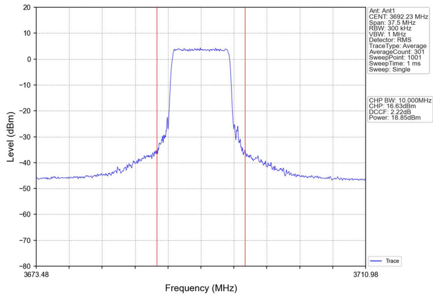
Band48_15MHz_QPSK_HCH_3692.5MHz_RB_36_39_NTNV
