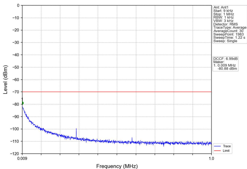
n48_30kHz_SISO_NTNV_10MHz_CP-OFDM QPSK_3555MHz_Inner_1RB_Left
