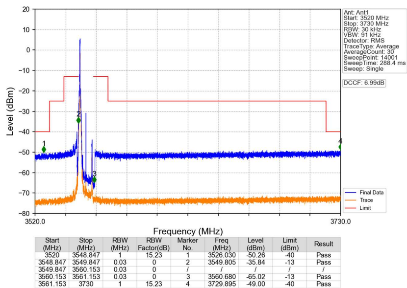
n48_30kHz_SISO_NTNV_10MHz_CP-OFDM QPSK_3555MHz_Edge_1RB_Left
