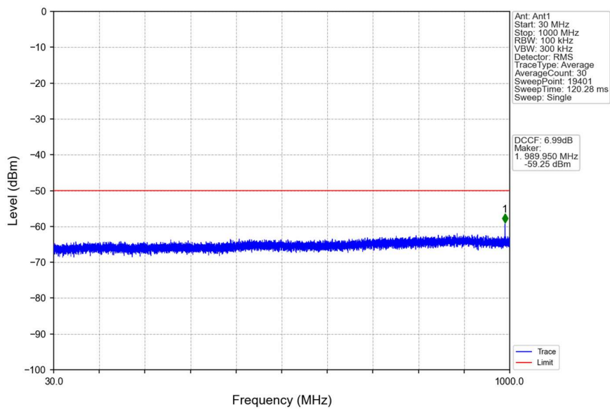
n48_30kHz_SISO_NTNV_10MHz_DFT-s-OFDM QPSK_3555MHz_Inner_1RB_Left
