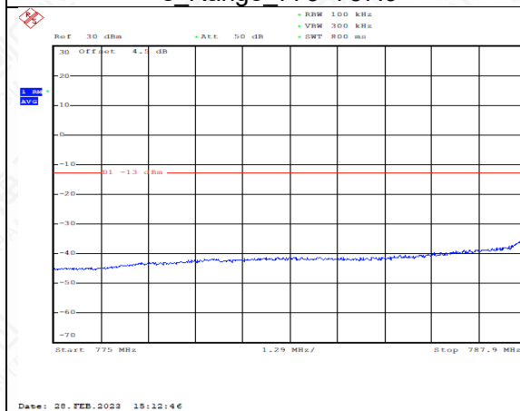
FDD14_10MHz_793_QPSK_fullRB_ExtraBand s_Range_775~787.9
