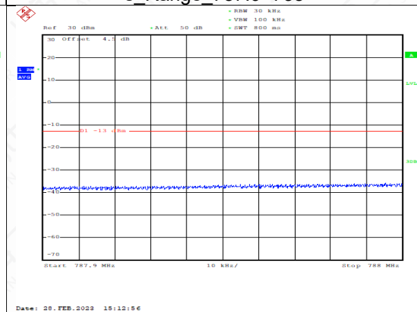
FDD14_10MHz_793_QPSK_fullRB_ExtraBand s_Range_787.9~788
