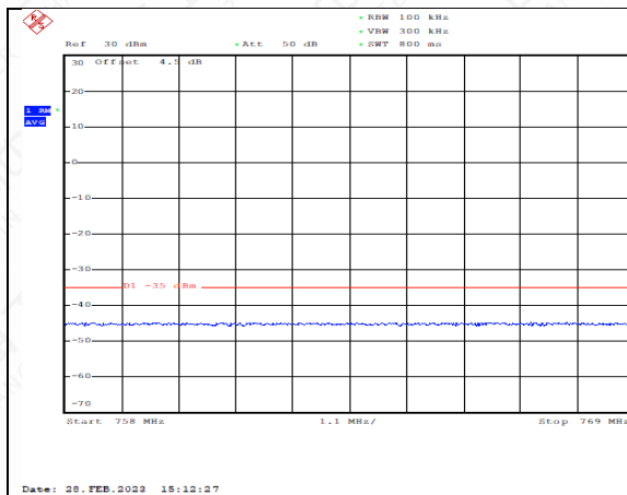
FDD14_10MHz_793_QPSK_fullRB_ExtraBand s_Range_758~769.9
