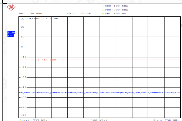
FDD14_10MHz_793_QPSK_OneRB_high_ExtraBands_Range_757~758
