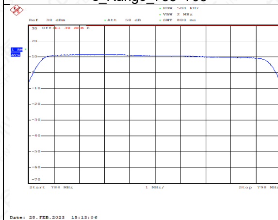
FDD14_10MHz_793_QPSK_fullRB_ExtraBand s_Range_788~798
