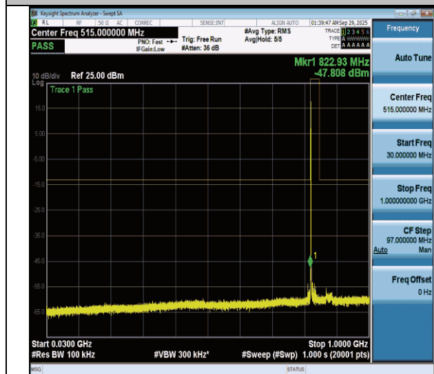
NTNV-n26(824-849)-PC3-15-20-L-CP-QPSK-Edge_1RB_Left-30- 1000-PASS
