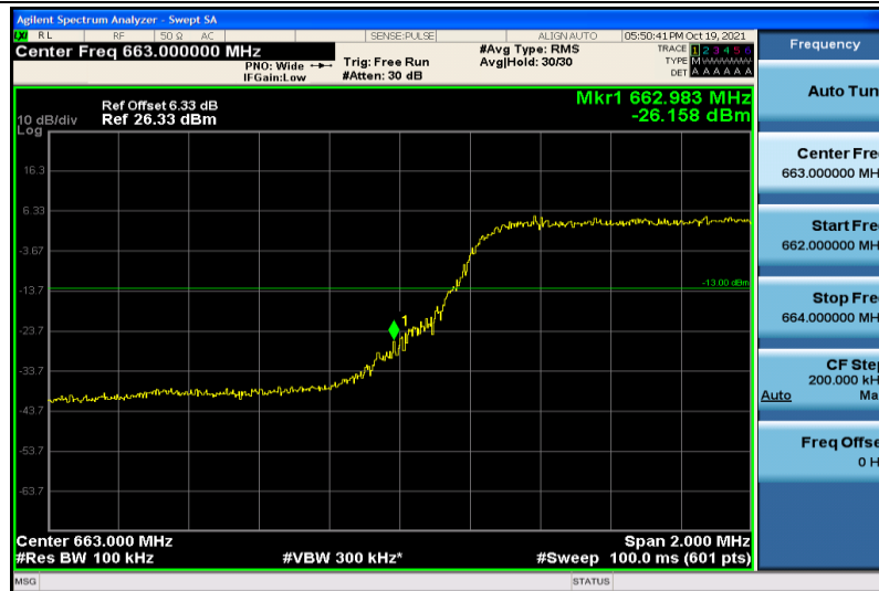
Band71-5MHz-QPSK-133147-25RB#0
