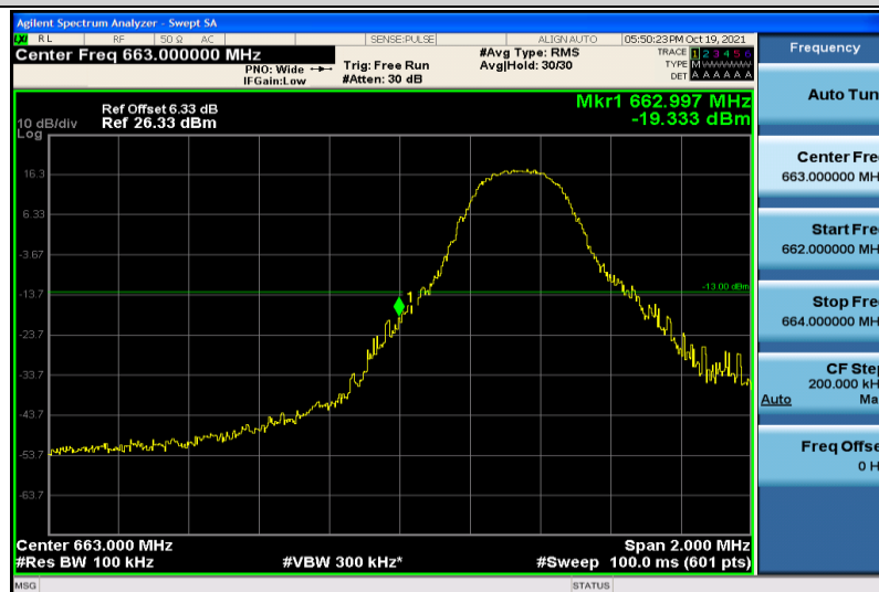
Band71-5MHz-QPSK-133147-1RB#0
