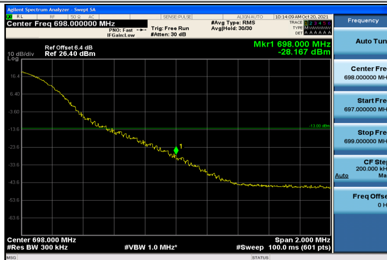
Band71-20MHz-QPSK-133372-1RB#99
