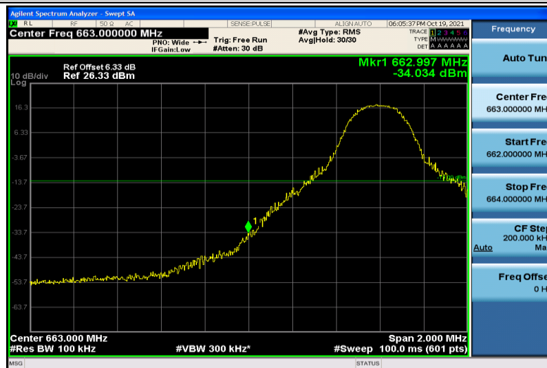
Band71-10MHz-QPSK-133172-1RB#0
