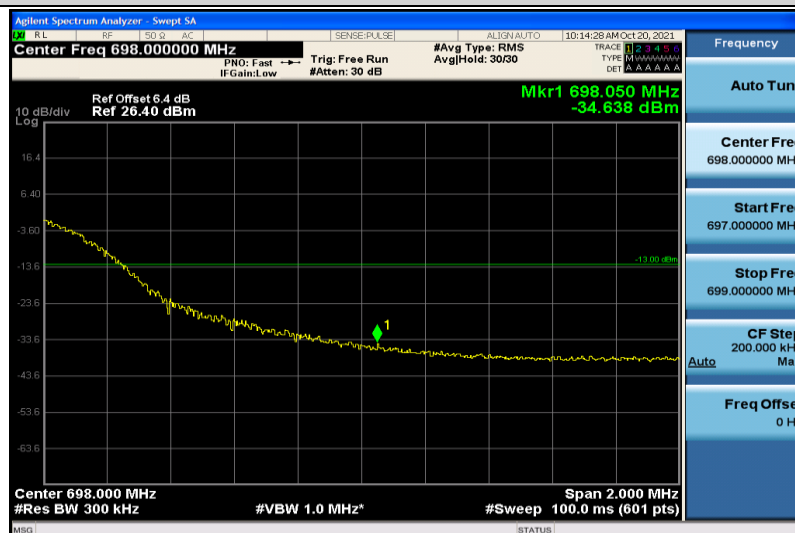
Band71-20MHz-QPSK-133372-100RB#0
