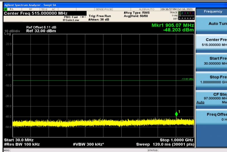
Band4-20MHz-QPSK-20300-1RB#0-30~1000MHz
