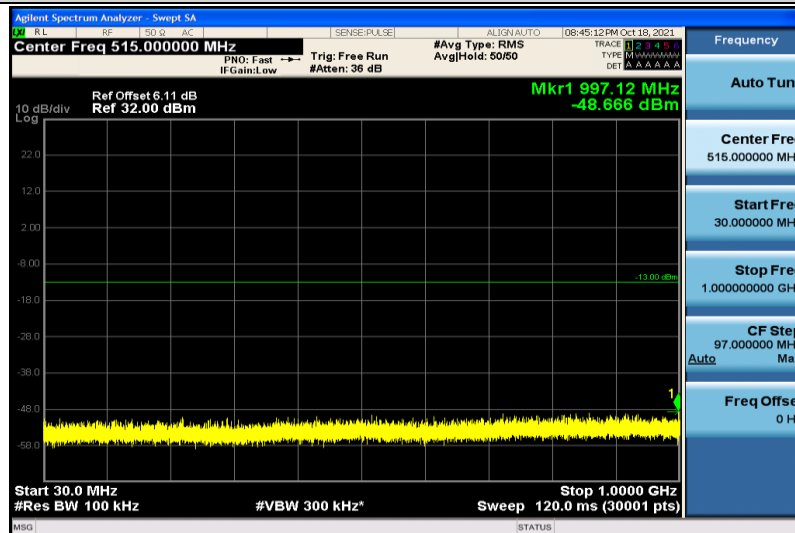
Band2-20MHz-16QAM-19100-1RB#0-30~1000MHz
