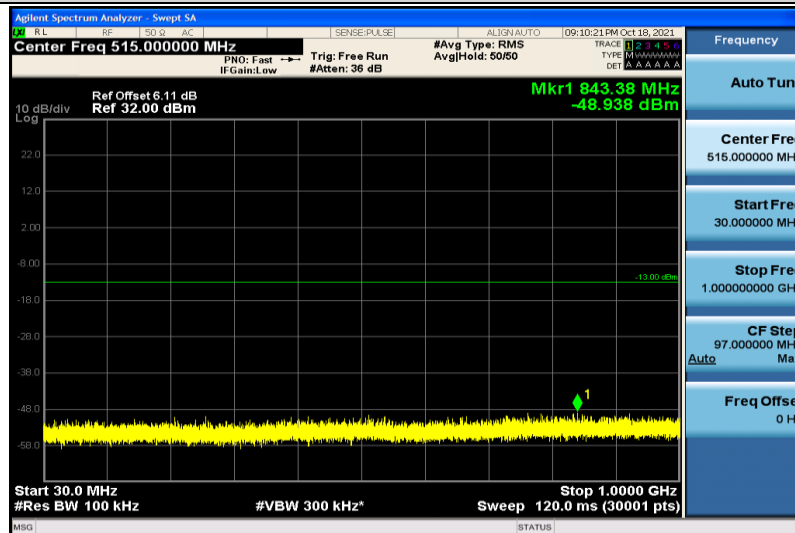
Band4-5MHz-QPSK-20375-1RB#0-30~1000MHz
