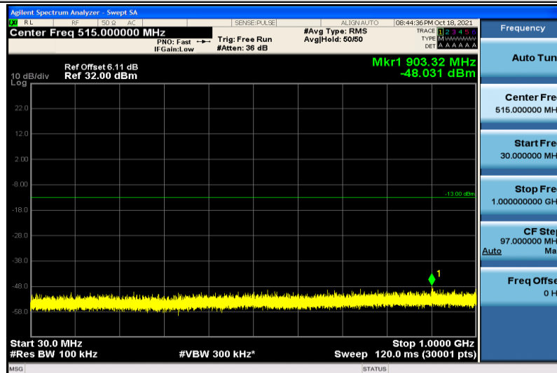
Band2-20MHz-QPSK-19100-1RB#0-30~1000MHz
