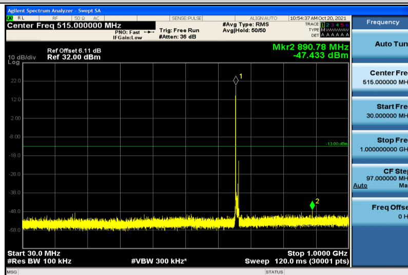
Band71-10MHz-QPSK-133172-1RB#0-30~1000MHz
