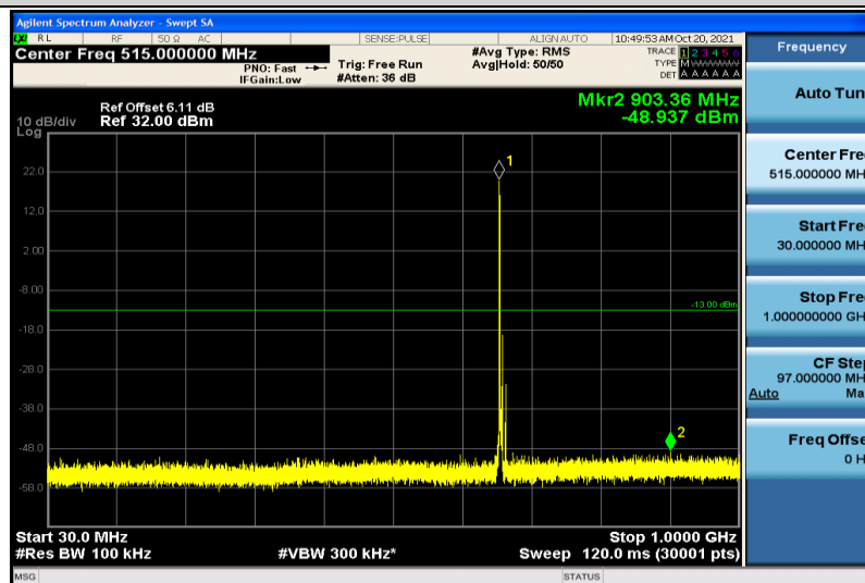
Band71-5MHz-QPSK-133147-1RB#0-30~1000MHz
