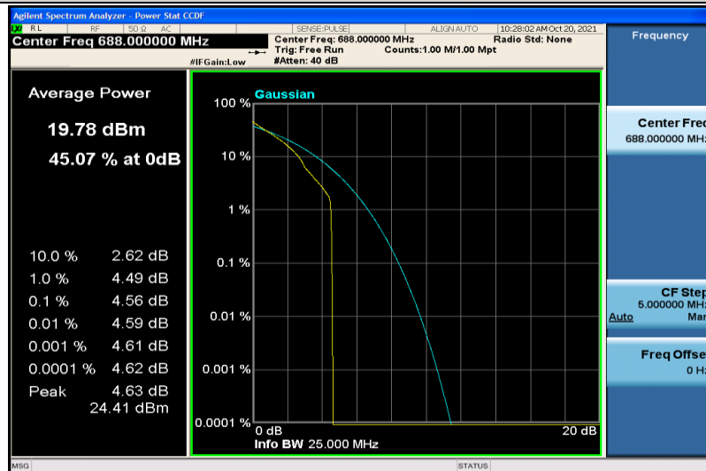
Band71-20MHz-QPSK-133372-1RB#0
