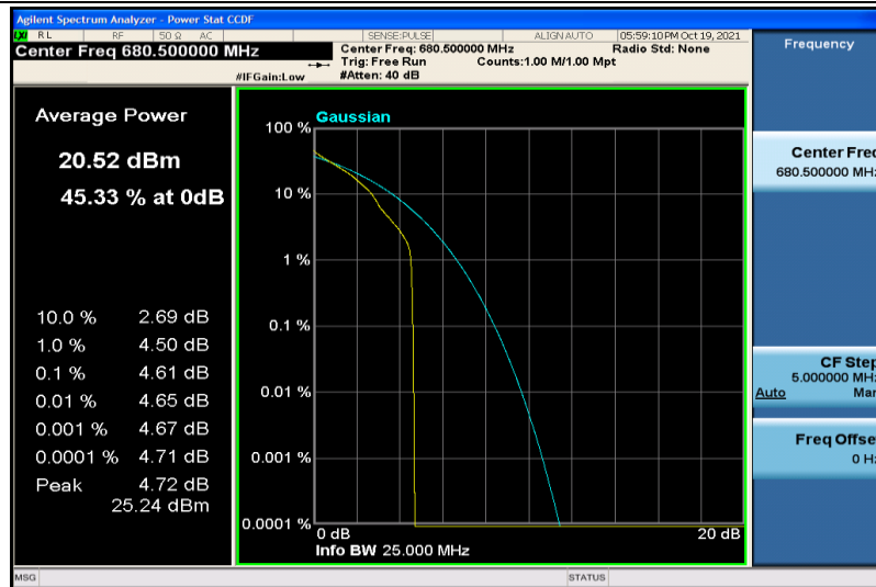
Band71-5MHz-QPSK-133297-1RB#0
