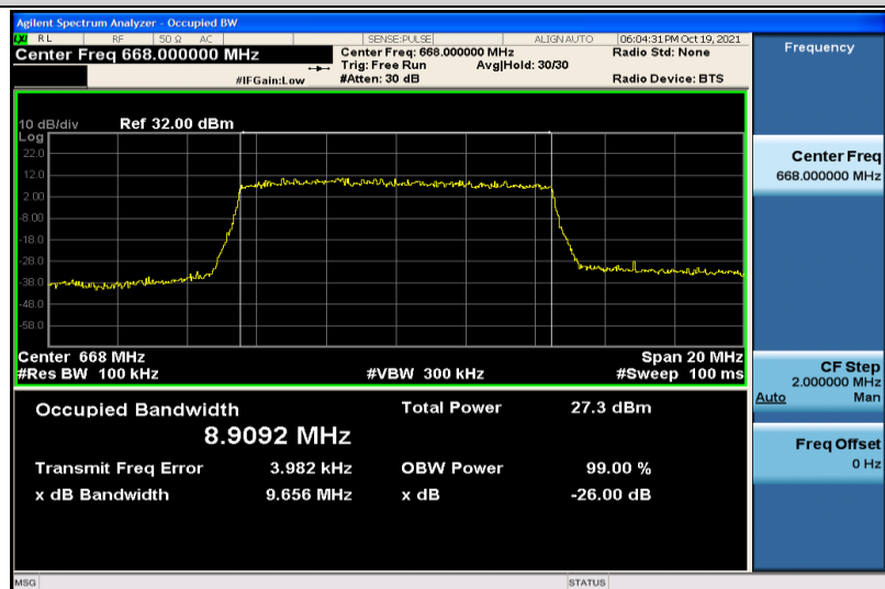
Band71-10MHz-QPSK-133172-50RB#0-8.9092
