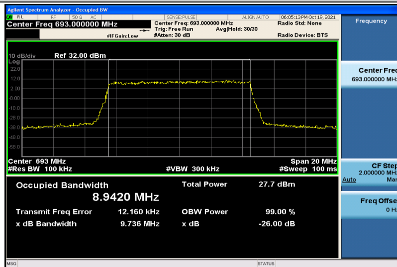
Band71-10MHz-QPSK-133422-50RB#0-8.9420
