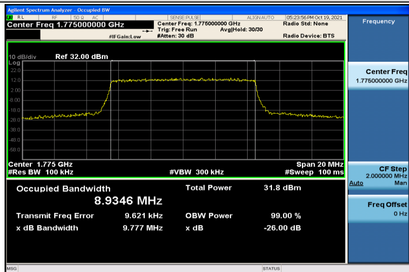
Band66-10MHz-QPSK-132622-50RB#0-8.9346
