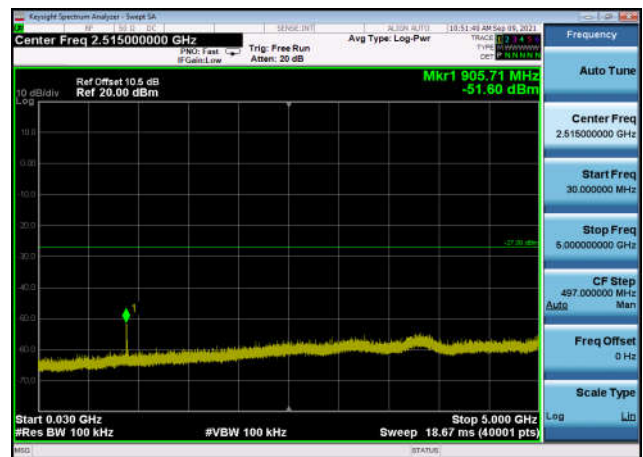
U-NII-2a ,Plot 2,30MHz~5000MHz-802.11ac(20MHz),5300MHz,Ant1
