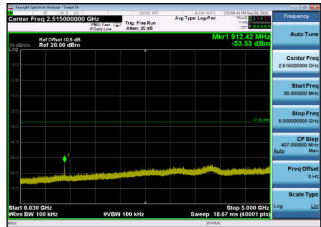
U-NII-2a ,Plot 2,30MHz~5000MHz-802.11 ac(80MHz),5290MHz,Ant1
