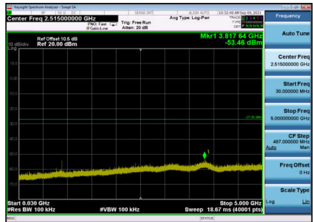
U-NII-2a ,Plot 2,30MHz~5000MHz-802.11a(20MHz),5320MHz,Ant1
