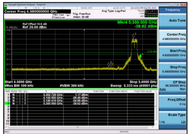
U-NII-2a ,Plot 1,Band Edge-802.11ac(40 MHz),5310MHz,Ant1
