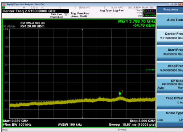
U-NII-2a ,Plot 2,30MHz~5000MHz-802.11 ac(40MHz),5310MHz,Ant1
