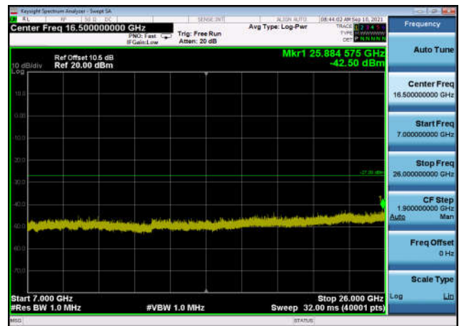
U-NII-2c ,Plot 4,7000MHz~26000MHz-802 .11ac(80MHz),5530MHz,Ant1
