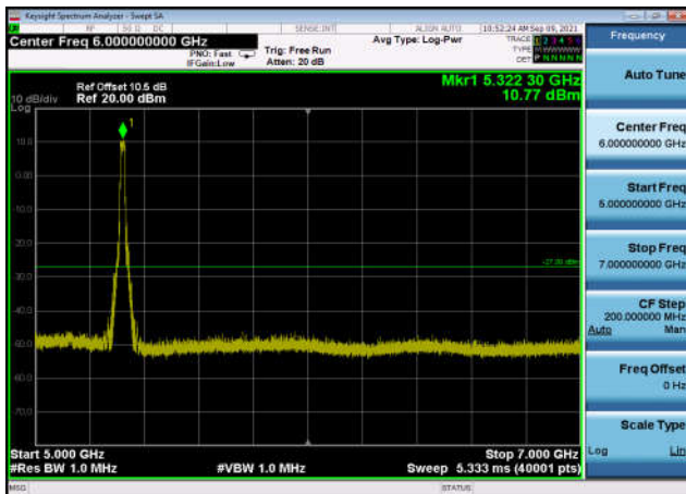
U-NII-2a ,Plot 3,5000MHz~7000MHz-802. 11ac(20MHz),5300MHz,Ant1
