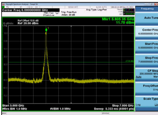
U-NII-2c ,Plot 3,5000MHz~7000MHz-802. 11ac(20MHz),5600MHz,Ant1
