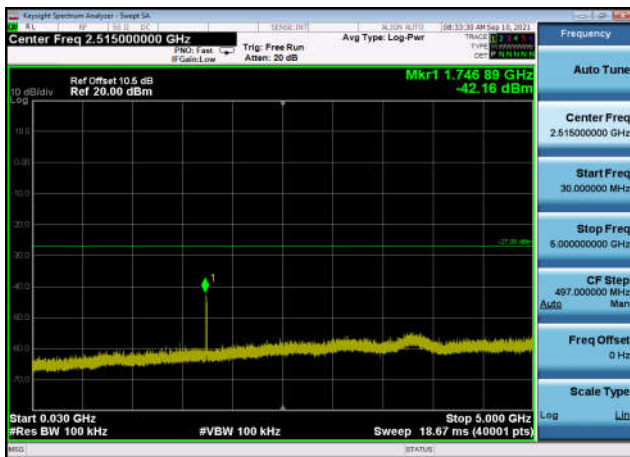
U-NII-2c ,Plot 2,30MHz~5000MHz-802.11 ac(40MHz),5670MHz,Ant1
