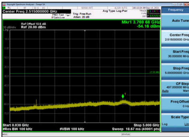
U-NII-2c ,Plot 2,30MHz~5000MHz-802.11 ac(20MHz),5700MHz,Ant1
