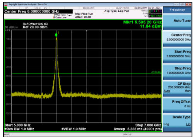
U-NII-2c ,Plot 3,5000MHz~7000MHz-802. 11ac(20MHz),5500MHz,Ant1
