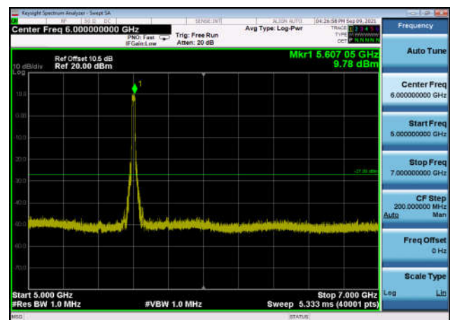
U-NII-2c ,Plot 3,5000MHz~7000MHz-802.11n(20MHz),5600MHz,Ant1
