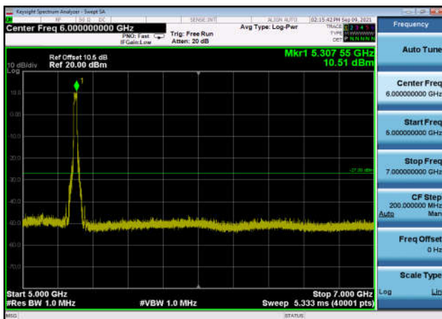
U-NII-2a ,Plot 3,5000MHz~7000MHz-802. 11ac(40MHz),5270MHz,Ant1
