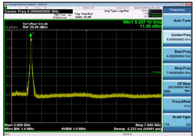
U-NII-2a ,Plot 3,5000MHz~7000MHz-802. 11ac(20MHz),5320MHz,Ant1
