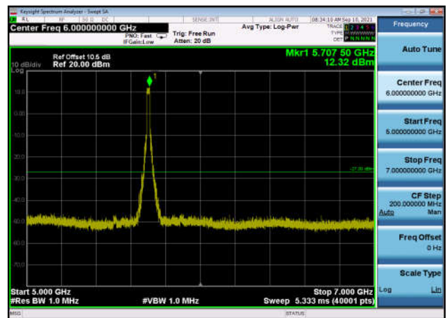
U-NII-2c ,Plot 3,5000MHz~7000MHz-802. 11ac(20MHz),5700MHz,Ant1
