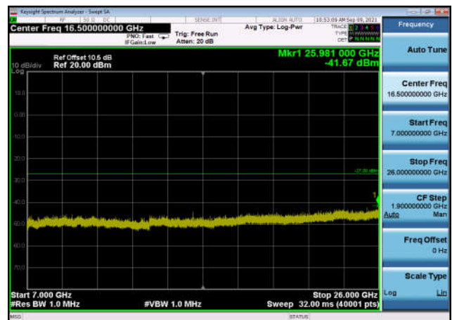
U-NII-2a ,Plot 4,7000MHz~26000MHz-802 .11ac(20MHz),5300MHz,Ant1
