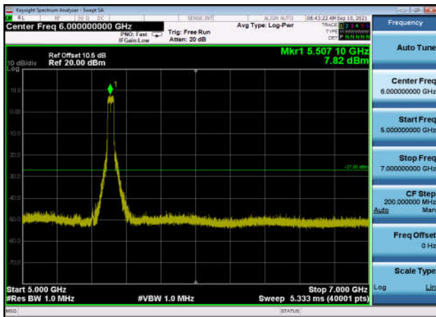
U-NII-2c ,Plot 3,5000MHz~7000MHz-802. 11ac(80MHz),5530MHz,Ant1
