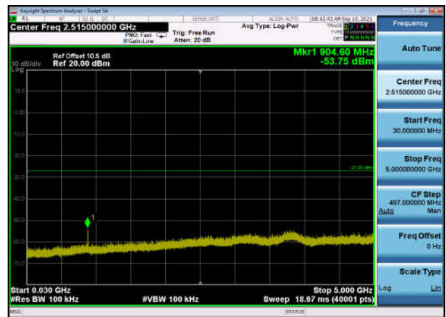
U-NII-2c ,Plot 2,30MHz~5000MHz-802.11 ac(80MHz),5530MHz,Ant1
