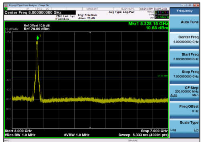
U-NII-2a ,Plot 3,5000MHz~7000MHz-802. 11ac(40MHz),5310MHz,Ant1
