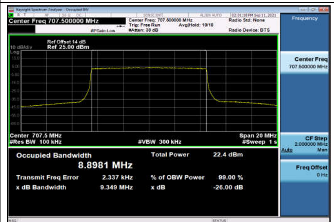
FDD12_MidRange_10_707.5_Q16
