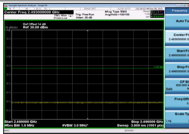
FDD07_10MHz_2505_Q16_OneRB_low _ExtraBands_Range_2490~2496
