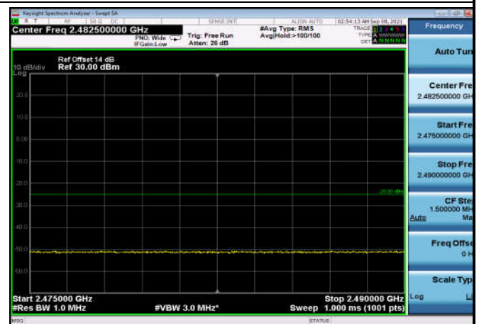
FDD07_20MHz_2510_Q16_fullRB_ExtraBand s_Range_2475~2490
