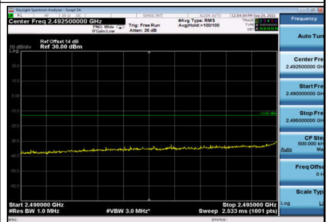
TDD41_10MHz_2501_Q16_FullRB_Low _ExtraBands_Range_2490~2495
