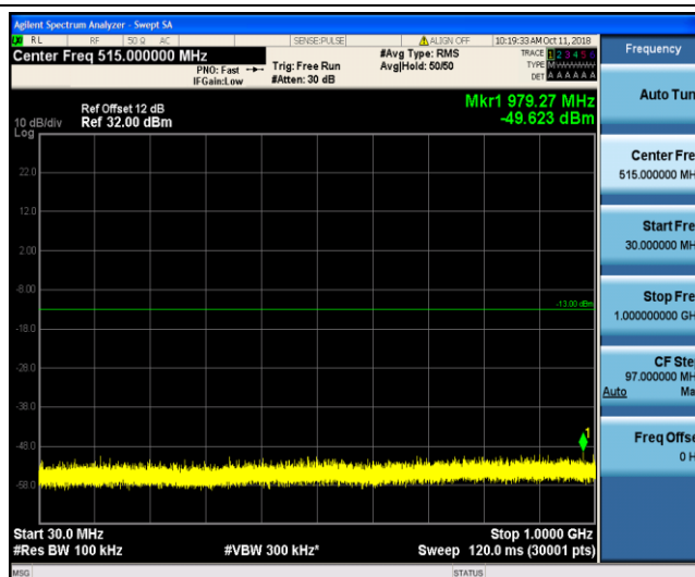
Band2 15MHz QPSK 18675 1RB#0
